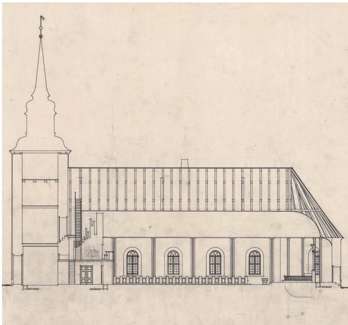
Fig. 18b. Forslag til kirkens ombygning, tegnet af Andreas Jensen 1947 (s. 1545). 1:300. Længdesnit set mod nord. I Danmarks Kunstbibliotek. – Proposal for rebuilding of church, drawn by Andreas Jensen, 1947. Longitudinal section looking north.
