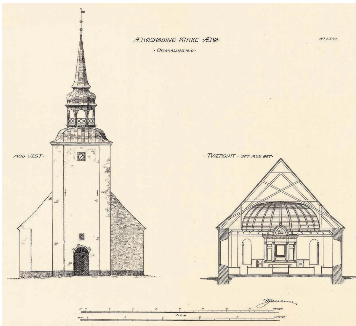
Fig. 14a. Opstalt af vestfacade og tværsnit set mod øst. 1:300. Målt og tegnet af Niels Jacobsen 1910. Aftryk i NM. – Elevation of west facade and cross-section looking east.
