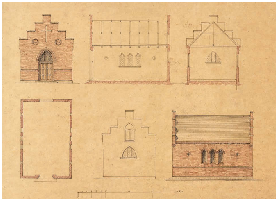
Fig. 10. Ikke anvendt forslag til ligkapel fra 1879 (s. 1534). 1:300. I NM. – Unrealized proposal for a mortuary chapel from 1879.
