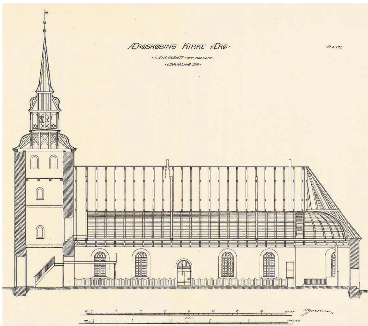
Fig. 14c. Længdesnit set mod nord. 1:300. Målt og tegnet af Niels Jacobsen 1910. Aftryk i NM. – Longitudinal section looking north.
