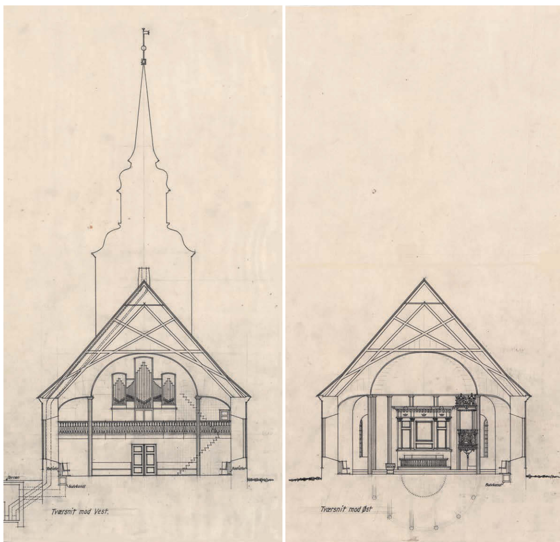
Fig. 18c-d. Forslag til kirkens ombygning, tegnet af Andreas Jensen 1947 (s. 1545). 1:300. Tværsnit set mod vest og øst. I Danmarks Kunstbibliotek. – Proposal for rebuilding of church, drawn by Andreas Jensen, 1947. Cross-section looking west and east.
