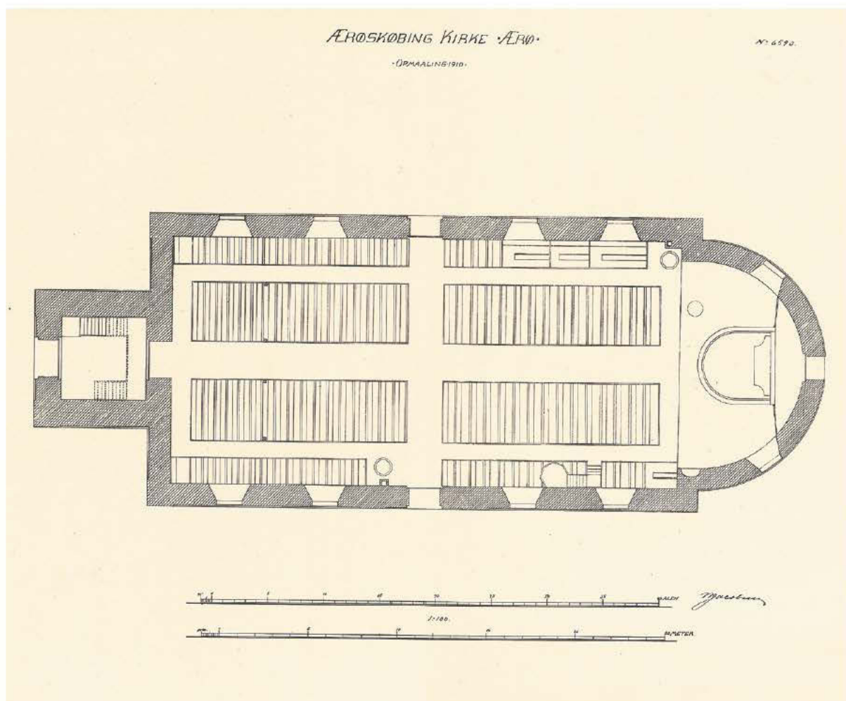
Fig. 14d. Grundplan. 1:300. Målt og tegnet af Niels Jacobsen 1910. Aftryk i NM. – Ground plan.
