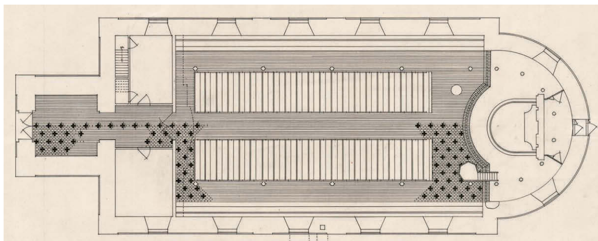
Fig. 17. Grundplan med forslag til bl.a. ny gulvbelægning, tegnet af Andreas Jensen 1949 (s. 1546). 1:300. I Danmarks Kunstabibliotek. – Ground plan with proposal for new flooring drawn by Andreas Jensen, 1949.
