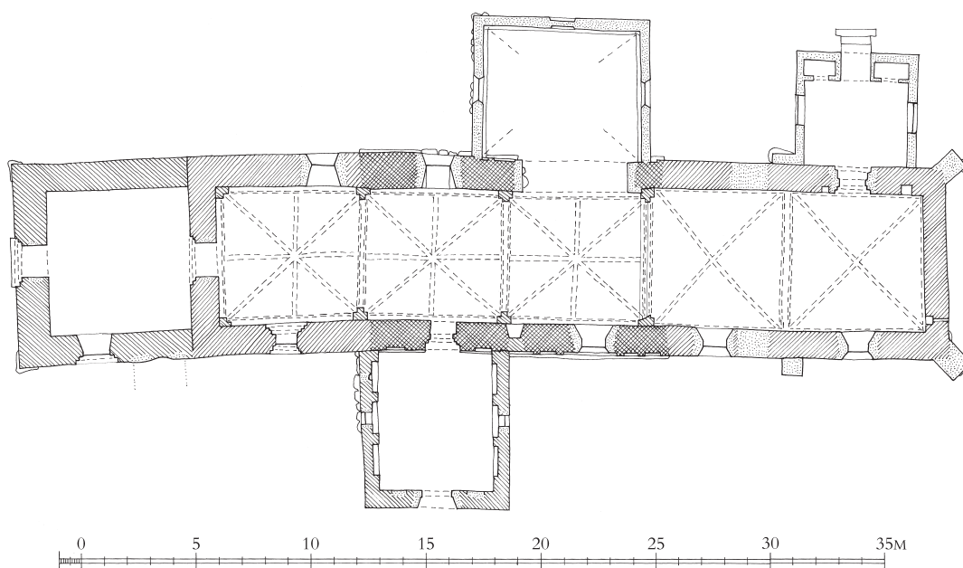
Fig. 9. Grundplan. 1:300. Målt af E. Mindedal Rasmussen 1951, suppleret af Pia K. Lindholt og tegnet af Thomas Bertelsen 2018. Signaturforklaring s. 9. – Ground plan. Key on p. 17.
