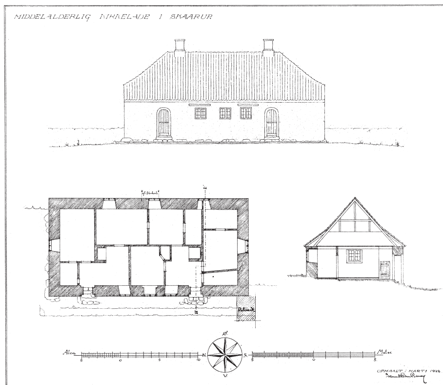
Fig. 5. Opstalt af østfacade, plan og tværsnit af kirkeladen med indretning som hospital (s. 1745). 1:300. Målt og tegnet af Knud Lehn Petersen 1922. I NM. – Elevation of east facade, plan and cross-section of the tithe barn with disposition as a hospital.
