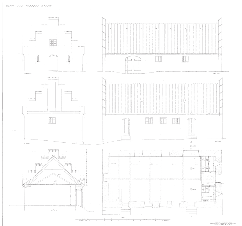
Fig. 107. Opstalt af facader, plan og tværsnit af kirkeladen med forslag til ny indretning (s. 1745). 1:300. Målt og tegnet af D. Rasmussen og E. Mindedal Rasmussen 1931. I NM. – Elevation of facades, plan and cross-section of the tithe barn with suggested new disposition.
