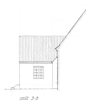
Fig. 12a-c. Opstalter. 1:300. a. Sydfacade. b. Østfacade. c. Vestfacade af sakristi (snit b-b). Målt og tegnet af E. Mindedal Rasmussen 1951. I NM. — Elevations. a. South facade. b. East facade. c. West facade of sacristy.
