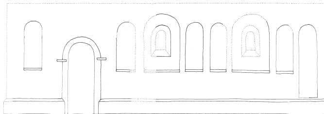
Fig. 11. Rekonstruktion af skibets romanske facadedekoration set mod nord (s. 1749). 1:150. Målt af E. Mindedal Rasmussen 1951, suppleret af Pia K. Lindholt og Anders C. Christensen, tegnet af Thomas Bertelsen 2018. – Reconstruction of the Romanesque facade decoration of the nave, looking north.
