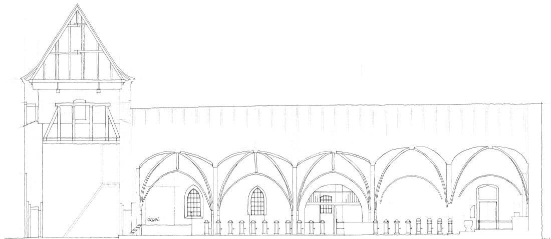
længdesnit
