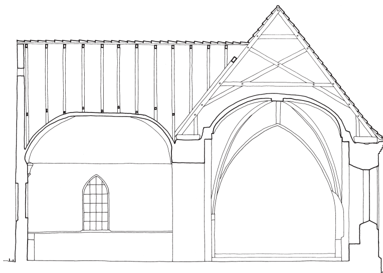
Fig. 8. Tværsnit. 1:150. Målt af E. Mindedal Rasmussen 1951, suppleret af Pia K. Lindholt og Anders C. Christensen, tegnet af sidstnævnte 2018. – Cross-section.
