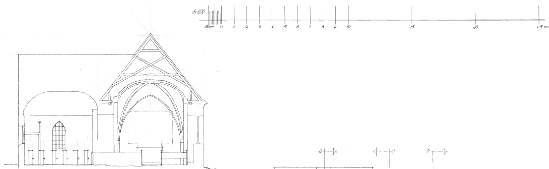
tværsnit a-a
