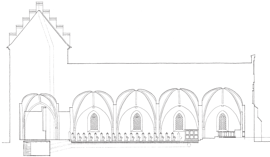
Fig. 6. Længdesnit set mod nord. 1:300. Målt og tegnet af Lars Mindedal 1992. I NM. – Longitudinal section looking north.
