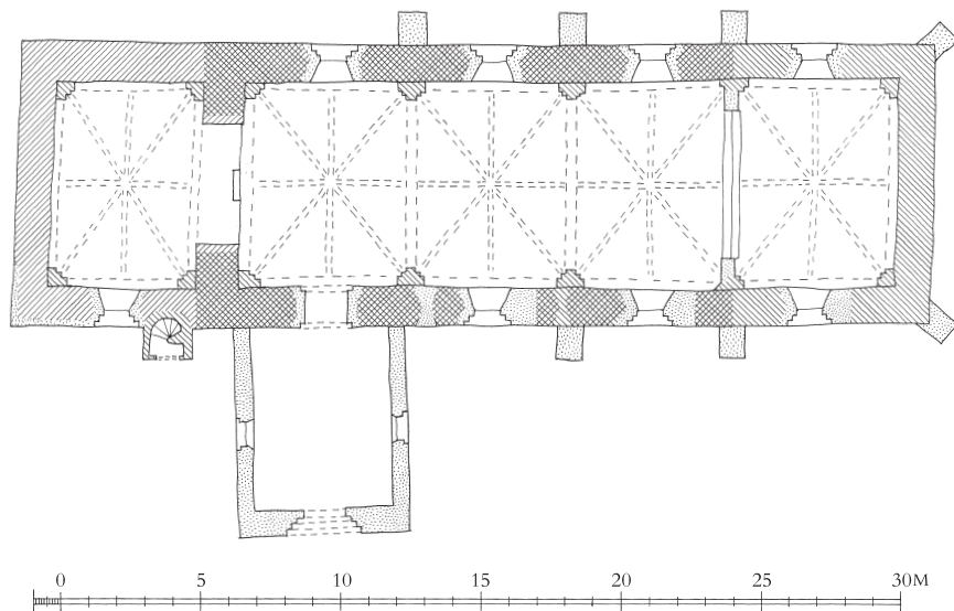
Fig. 7. Grundplan. 1:300. Efter opmåling af Lars Mindedal 1992, suppleret og tegnet af Pia K. Lindholt 2018. Signaturforklaring s. 9. – Ground plan. Key on p. 17.
