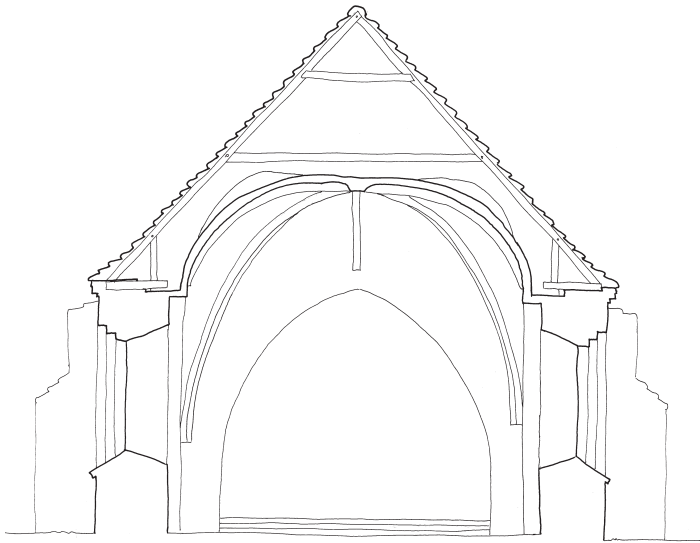
Fig. 5. Tværsnit. 1:150. Målt af Lars Mindedal 1991, suppleret af Anders C. Christensen og Pia K. Lindholt og tegnet af sidstnævnte 2018. – Cross-section.
