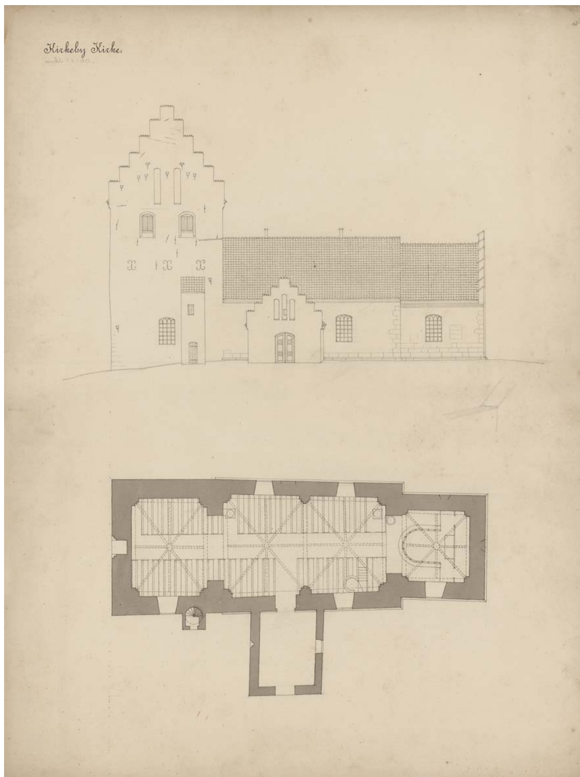
Fig. 16a-b. Opmålinger. 1:300. Målt og tegnet af J. Vilh. Petersen 1890. I NM. a. Opstalt af sydfacade. b. Grundplan. — a. Elevation of south facade. b. Ground plan.
