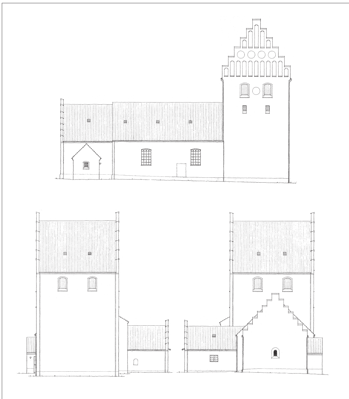
Fig. 23c-e. Opstalter. 1:300. Målt og tegnet af Lars Mindedal 1986. I NM. c. Nordfacade. d. Vestfacade. e. Østfacade. – Elevations. c. North facade. d. West facade. e. East facade.
