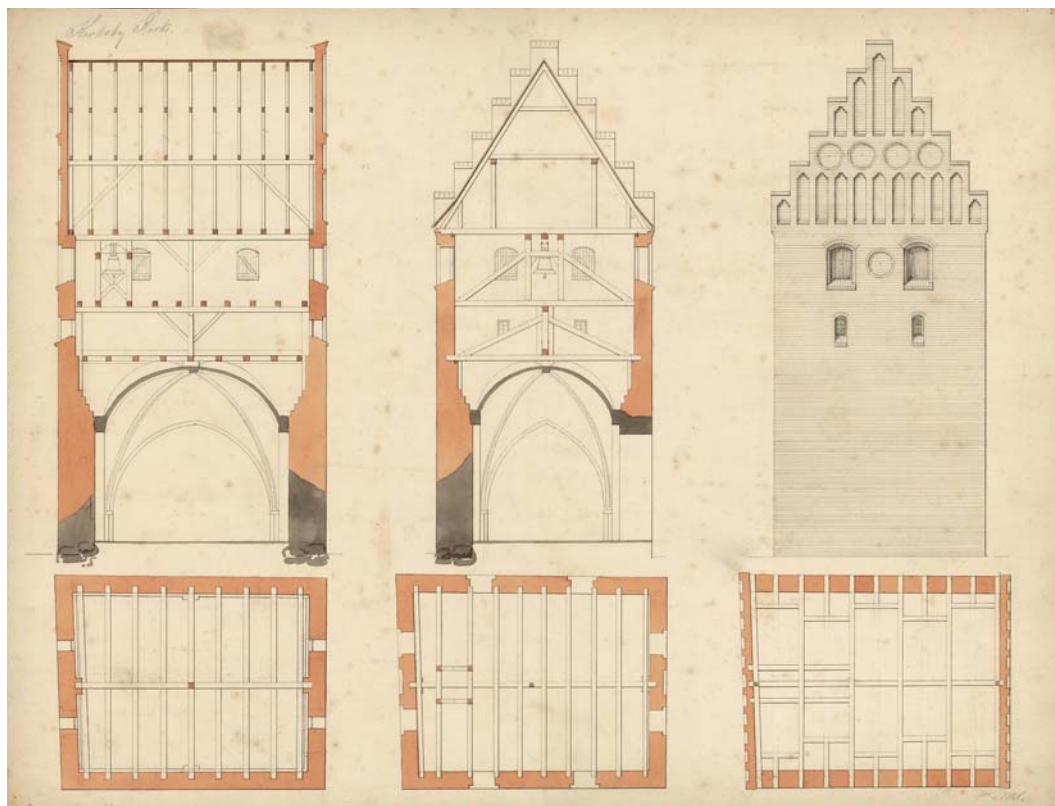
Fig. 17a-f. Ombygning af tårn (s. 2080), bevaret senmiddelalderligt murværk markeret med gråt. 1:300. Tegnet af J. Vilh. Petersen 1890. I NM. a. Snit set mod vest. b. Snit set mod nord. c. Opstalt af sydfacade. d. Plan af mellemstokværk. e. Plan af klokkestokværk. f. Plan af loftsrums. — The reconstructed tower with marking in grey of preserved Late Medieval masonry. a. Section looking west. b. Section looking north. c. Elevation of south facade. d. Plan of intermediate floor. e. Plan of belfry floor. f. Plan of loft.
