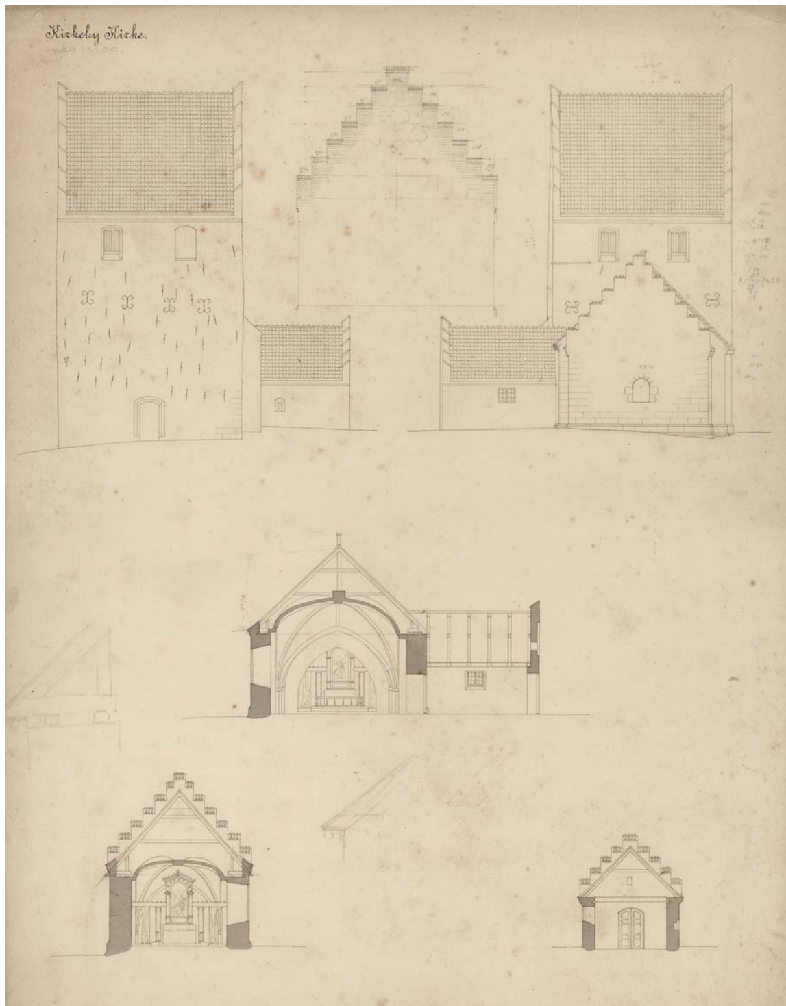
Fig. 16e-i. Opmålinger. 1:300. Målt og tegnet af J.Vilh. Petersen 1890. I NM. e. Opstalt af vestfacade. f. Opstalt af østfacade. g. Tværnsnit af skib og våbenhus set mod øst. h. Tværnsnit af kor set mod øst. i. Tværnsnit af våbenhus set mod syd. — e. Elevation of west facade. f. Elevation of east facade. g. Cross-section of nave looking east. h. Cross-section of chancel and porch looking east. i. Cross-section of porch looking south.
