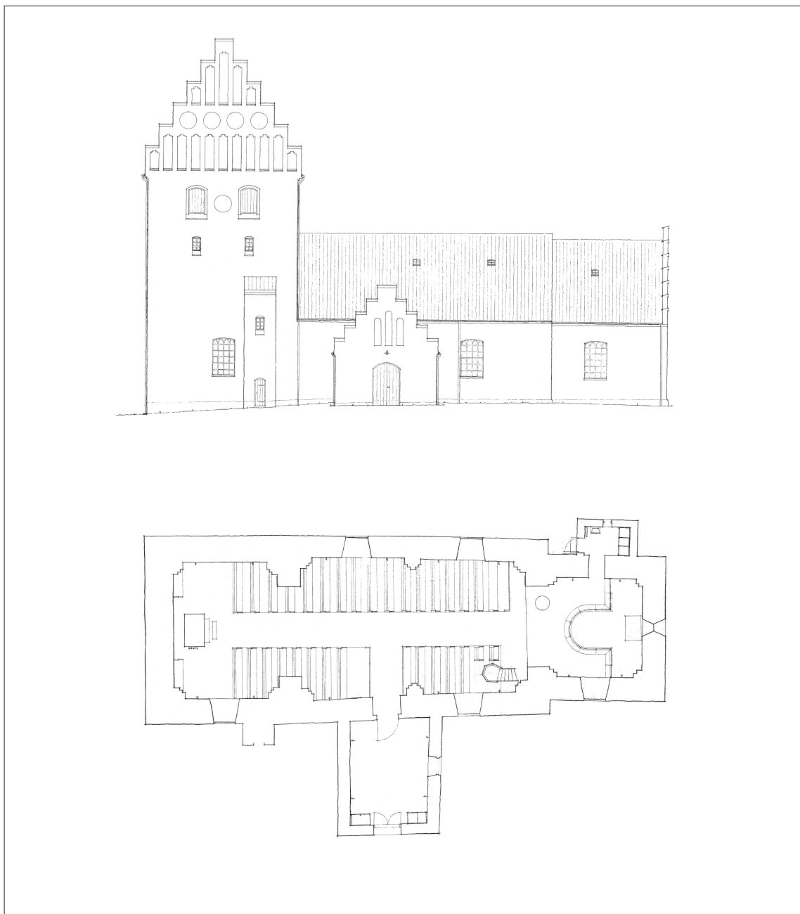
Fig. 23a-b Opstalt og plan. 1:300. Målt og tegnet af Lars Mindedal 1986 og 1974. I NM. a. Sydfacade. b. Plan. – Elevation and plan. a. South facade. b. Plan.
