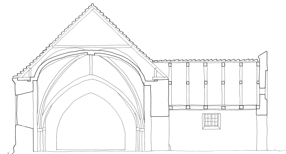
Fig. 6. Tværsnit. 1:150. Målt af J. Vilh. Petersen 1890, suppleret og tegnet af Pia K. Lindholt 2018. – Cross-section.
