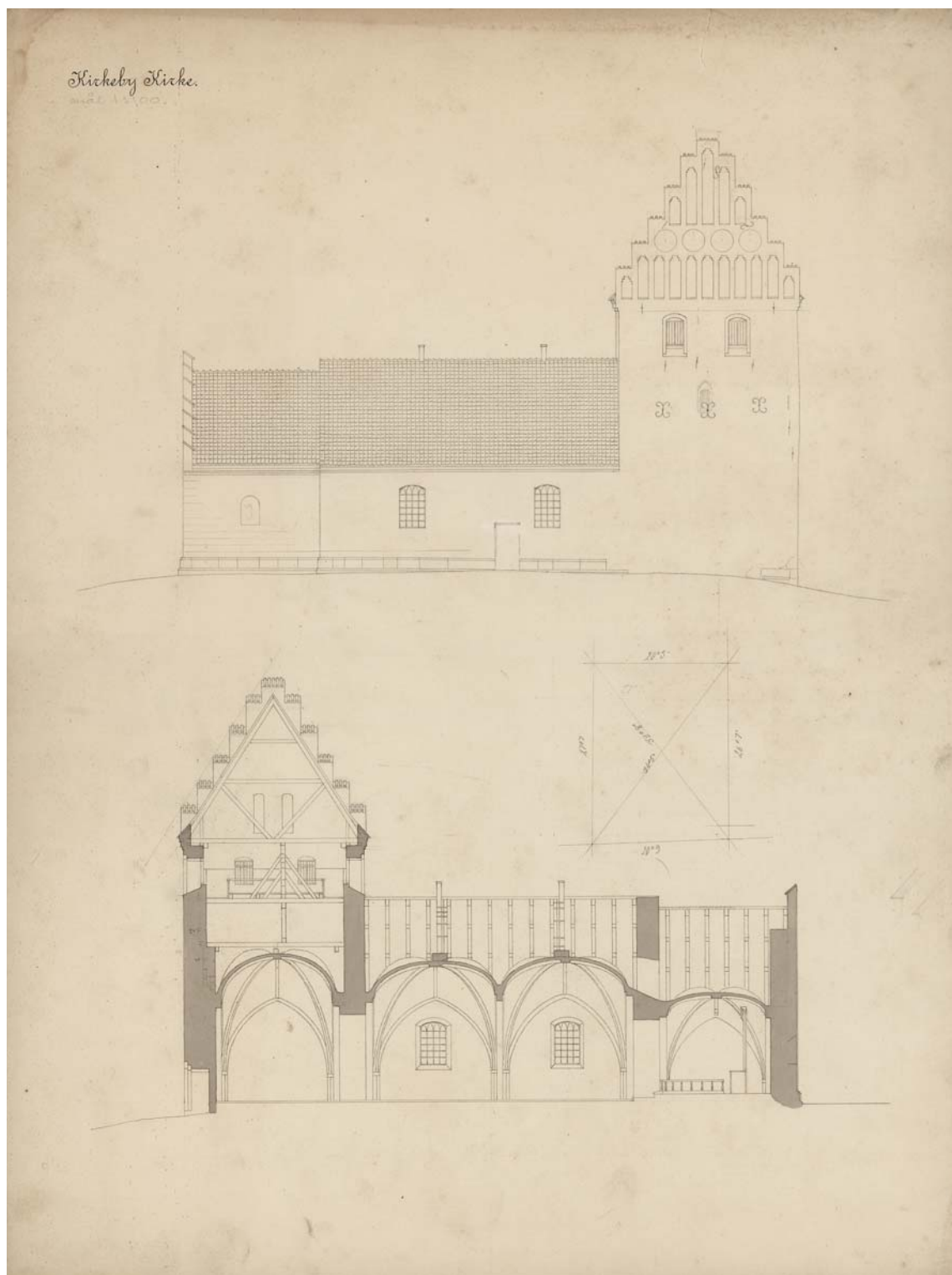
Fig. 16c-d. Opmålinger. 1:300. Målt og tegnet af J. Vilh. Petersen 1890. I NM. c. Opstalt af nordfacade. d. Længdesnit set mod nord. – c. Elevation of north facade. d. Longitudinal section looking north.
