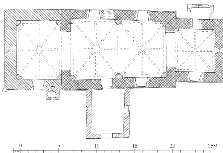
Fig. 7. Grundplan. 1:300. Efter opmåling af Lars Mindedal 1974, suppleret og tegnet af Pia K. Lindholt 2018. Signaturforklaring s. 9. – Ground plan. Key on p. 17.
