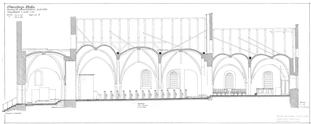
Fig. 10. Længdesnit set mod nord. 1:300. Målt og tegnet af Ejnar Mindedal Rasmussen 1955. I NM. – Longitudinal section looking north.
