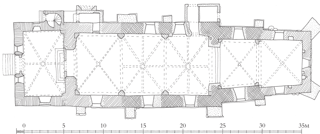
Fig. 8. Grundplan. 1:300. Efter opmåling af Ejnar Mindedal Rasmussen 1955, suppleret og tegnet af Pia K. Lindholt 2019. Signaturforklaring s. 9. – Ground plan. Key on p. 17.
