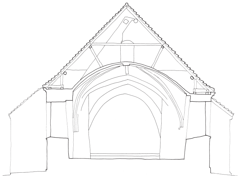
Fig. 7. Tværsnit. 1:150. Målt af Anders C. Christensen og Pia K. Lindholt og tegnet af sidstnævnte 2019. – Cross-section.
