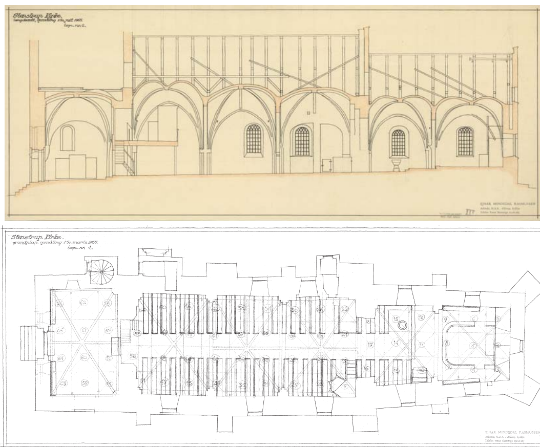
Fig. 77-78. 77. Længdesnit set mod nord. 78. Grundplan. 1:300. Målt og tegnet af Ejnar Mindedal Rasmussen 1955. I NM. – 77. Longitudinal section looking north. 78. Ground plan.
