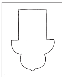
Fig. 81. Formsten i korforlængens hvælvribber (s. 2123). 1:10. Målt og tegnet af Pia K. Lindholt 2019. – Cross section of the ribs of the vaults in the chancel extension.
