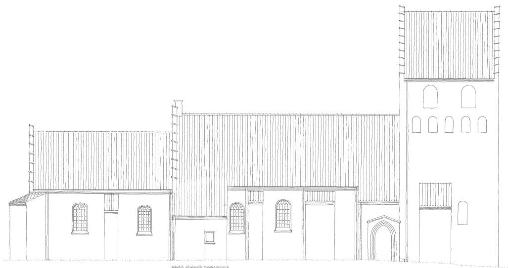
Fig. 9. Opstalt af nordfacade. 1:300. Målt og tegnet af Lars Mindedal 1960. I NM. – Elevation of north facade.
