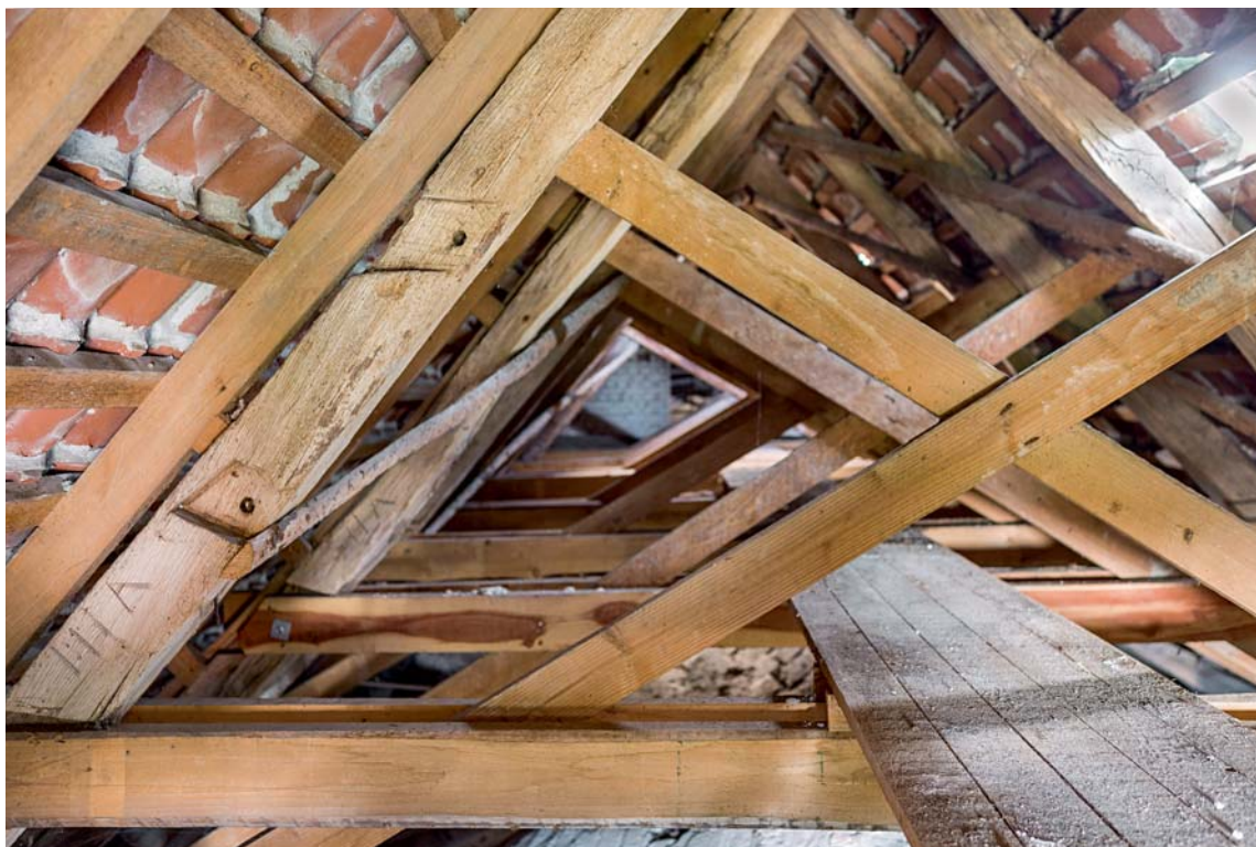
Fig. 23. Korets tagværk set mod vest (s. 2136). Foto Arnold Mikkelsen 2018. – Roofing of chancel looking west.
