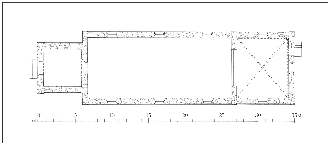
Fig. 4. Grundplan. 1:300. Målt af Ejnar Mindedal Rasmussen 1936, suppleret og tegnet af Pia K. Lindholt 2018. Signaturforklaring s. 9. – Ground plan. Key on p. 17.
