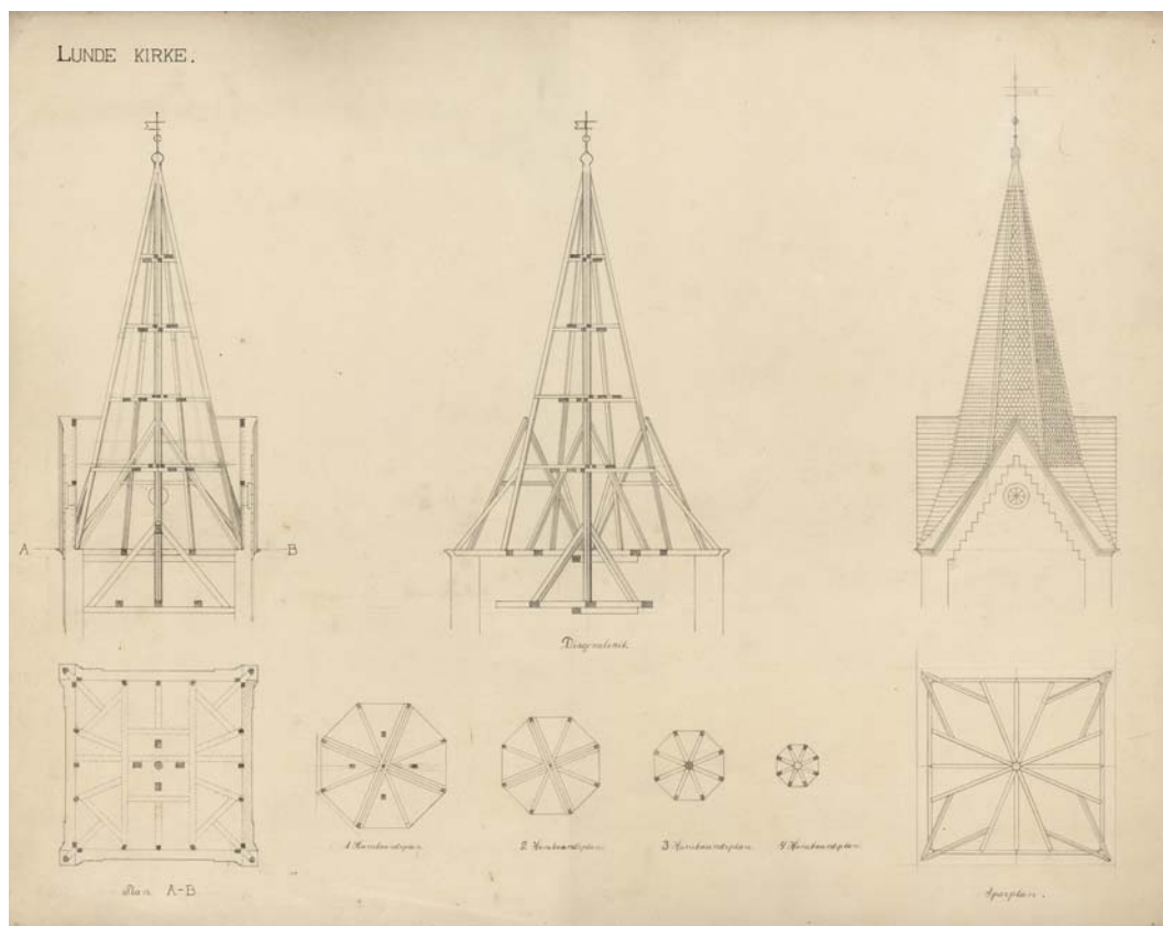
Fig. 7. Konstruktion af tårnets spir (s. 2192). 1:300. Tværsnit, diagonalsnit og opstalt; plan, 4 hanebåndsplæn samt spærplan. Opmåling o. 1885. I NM. – Construction of tower spire. Cross-section, diagonal section, exterior, plan, 4 tie beam plans and rafter plan.
