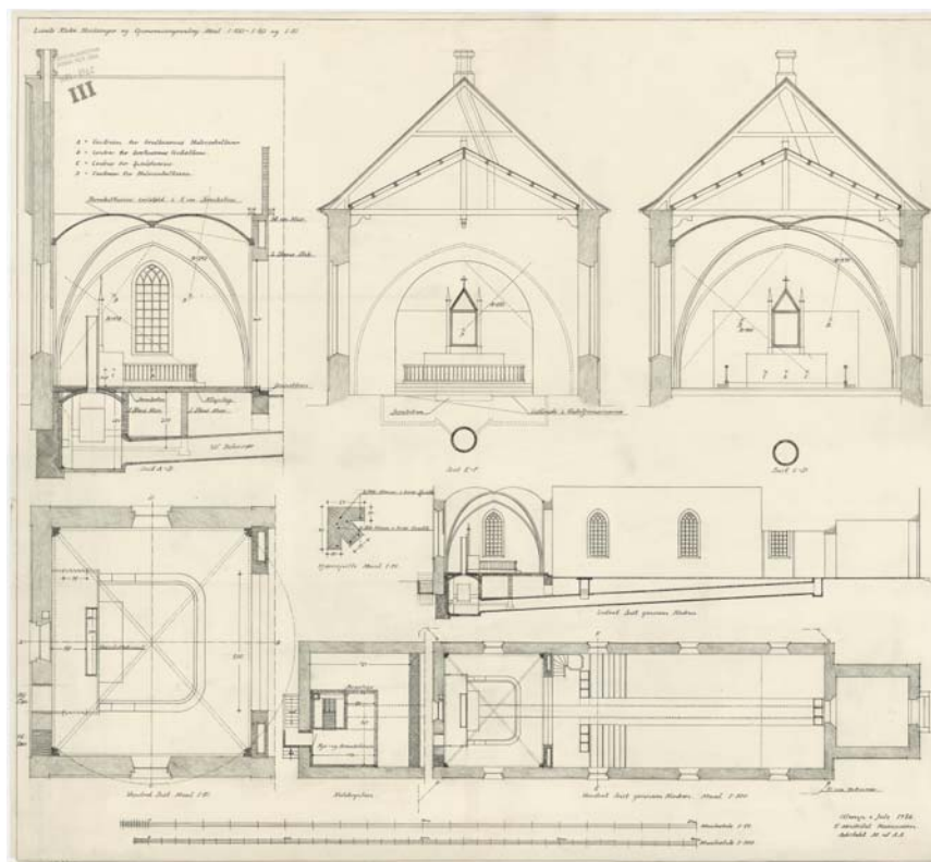
Fig. 8. Forslag til ombygning af kirkens kor (s. 2192). 1:300. Længdesnit af kor set mod syd, tværnsnit af skib set mod øst, tværskib af kor set mod øst samt plan af kor. Forslag til nyt varmeanlæg (s. 2194). 1:600. Længdesnit af kirken set mod syd, plan af fyrrkælder samt grundplan. Målt og tegnet af Ejnar Mindedal Rasmussen 1936. I NM. – Proposal for the rebuilding of the chancel of the church. 1:300. Longitudinal section of chancel looking south, cross-section of nave looking east and cross-section of chancel looking east. Proposal for a new heating system. 1:600. Longitudinal section of church looking south, plan of basement and ground plan of church.
