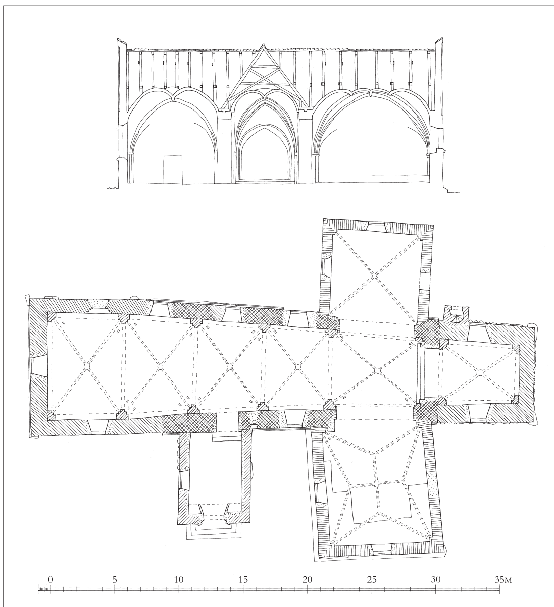
Fig. 10-11. 10. Tværsnit set mod øst. 1:300. Målt af Frits Bo Jørgensen 1959, suppleret og tegnet af Pia K. Lindholt 2019. 11. Grundplan. 1:300. Målt af C&W Arkitekter 2005, suppleret og tegnet af Pia K. Lindholt 2019. Signaturforklaring s. 9. – 10. Cross-section looking east. 11. Ground plan. Key on p. 17.
