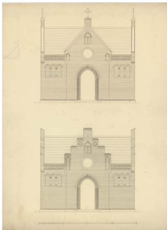
Fig. 4a-b. Opstalter af gravkapel på kirkegården (s. 2217). Vestfacade. 1:300. a. Oprindelig facade. b. Nuværende facade. Målt og tegnet J. Vilh. Petersen 1898. I NM. – Elevations of the sepulchral chapel in the churchyard. West facade. a. Original facade. b. Present facade.
