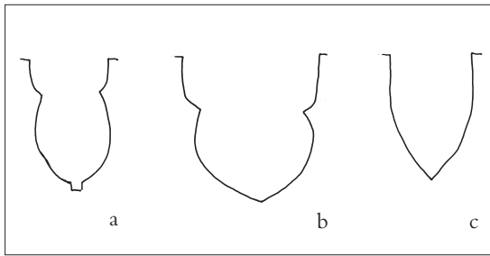
Fig. 164. Ribbeprofiler. 1:10. a. Skibets første fag. b. Skibets tredje og femte fag. c. Søndre og nordre korsarm. Målt af Thomas Bertelsen og Pia K. Lindholt, tegnet af sidstnævnte 2019. – Rib profiles. a. First bay of nave, b. Third and fifth bay of nave. c. South and north transepts.
