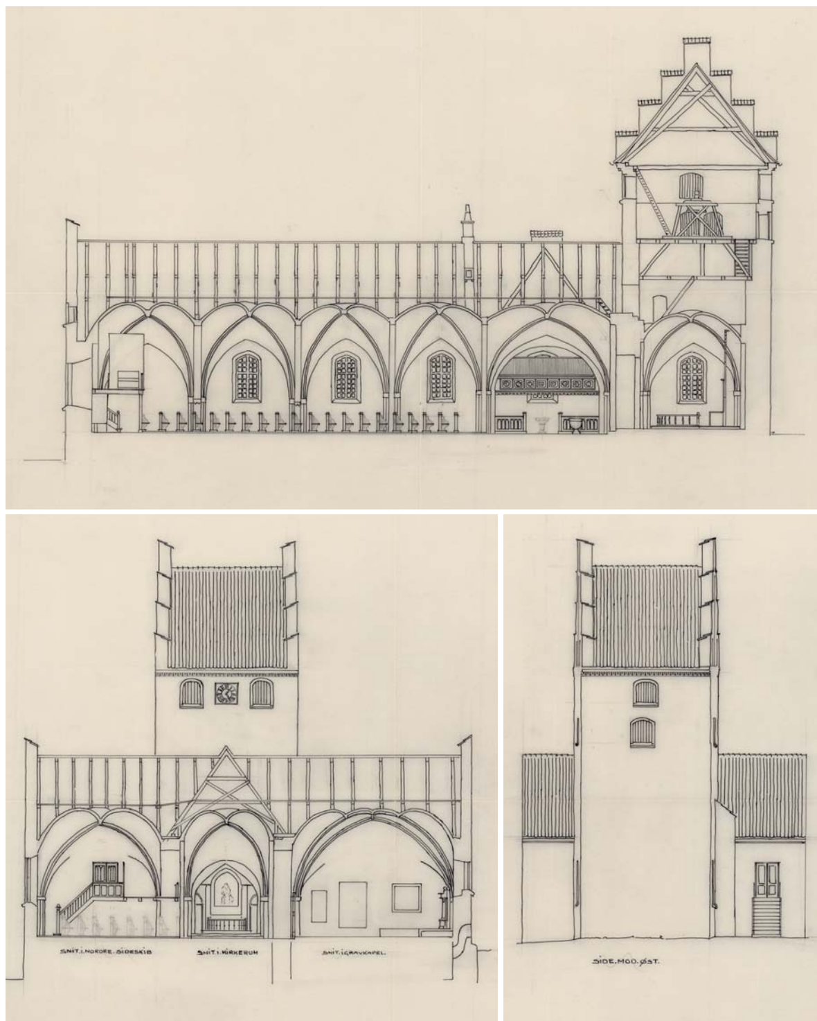
Fig. 36c-e. Opmålinger af kirken. 1:300. c. Længdesnit set mod nord. d. Tværsnit gennem skibets første fag og korsarmene set mod øst. e. Opstalt af østfacade. Målt og tegnet af Frits Bo Jørgensen 1959. I Danmarks Kunstbibliotek. — Scale drawings of the church. c. Longitudinal section looking east. d. Cross-section through the first bay of the nave and the transepts, looking east. e. Elevation of east facade.
