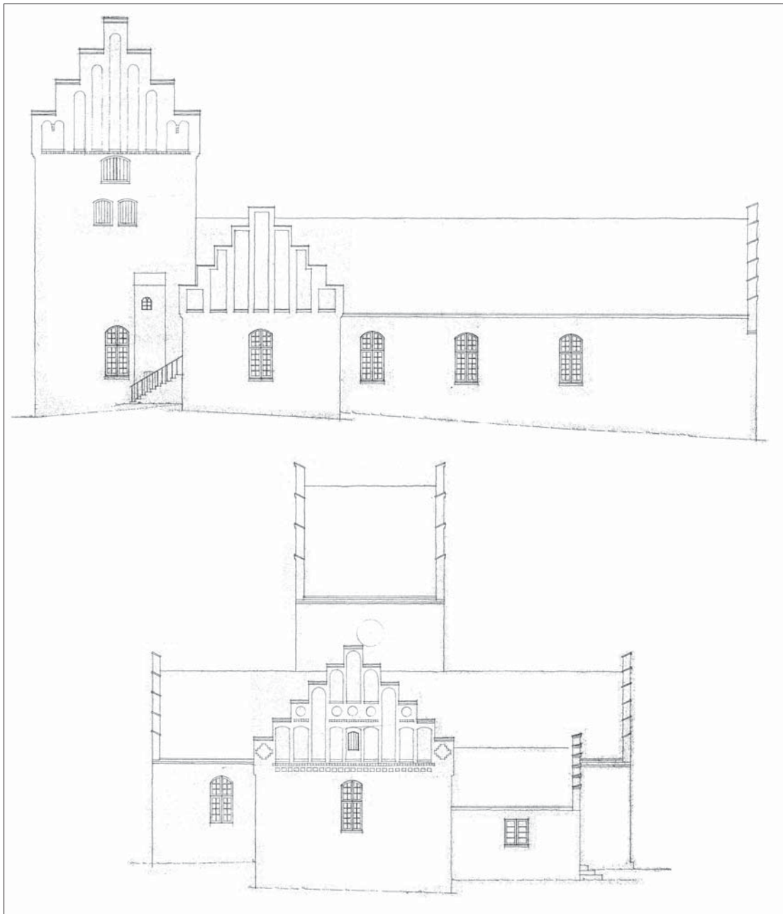
Fig. 12a-b. Opstalter af kirkens facader. 1:300. a. Nordfacade. b. Vestfacade. Målt og tegnet af Lars Mindedal 1974. Hos Rønnow Arkitekter. – Elevations of the church facades. a. North facade. b. West facade.
