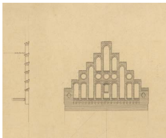
Fig. 38. Forslag til ny gavltrekanter på vestforlængelsen (s. 2244). 1:300. Usigneret tegning i NM. – Proposal for new pediment in the north wall of the western extension.
