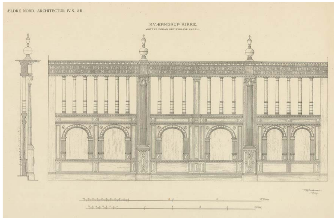
Fig. 104. Gitter, 1616, for Ulfeldts kapel (s. 2304). 1:50. Målt og tegnet af V. C. Christensen 1904. I NM (efter Tegninger af ældre nordisk Arkitektur , 1905). – Grating, 1616, for the Ulfeldt Chapel.
