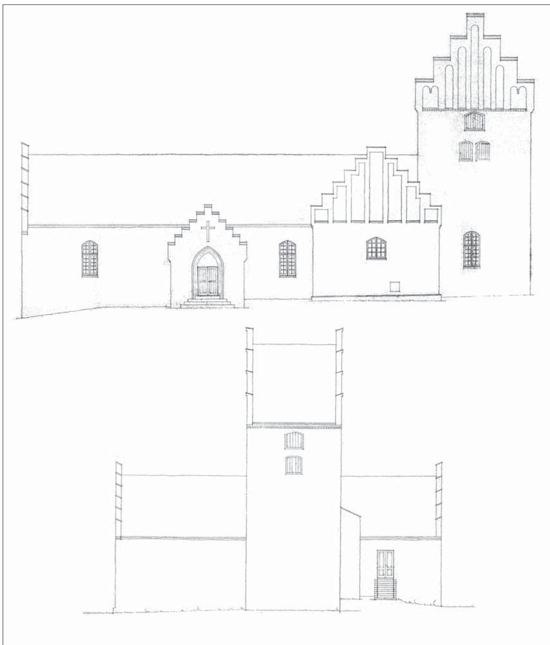
Fig. 12c-d. Opstalter af kirkens facader. 1:300. c. Sydfacade. d. Østfacade. Målt og tegnet af Lars Mindedal 1974. Hos Rønnow Arkitekter. – Elevations of the church facades. c. South facade. d. East facade.
