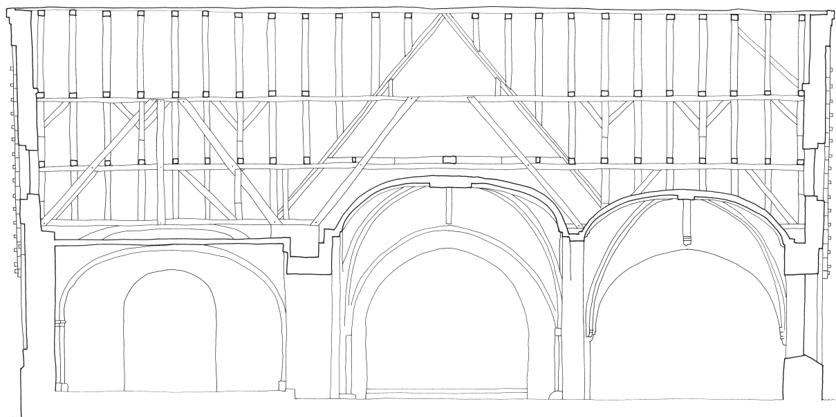
Fig. 9. Tværnsnit gennem skibets andet fag set mod øst. 1:150. Målt af Anders C. Christensen og Pia K. Lindholt, tegnet af sidstnævnte 2019. – Cross-section through the second bay of the nave looking east.
