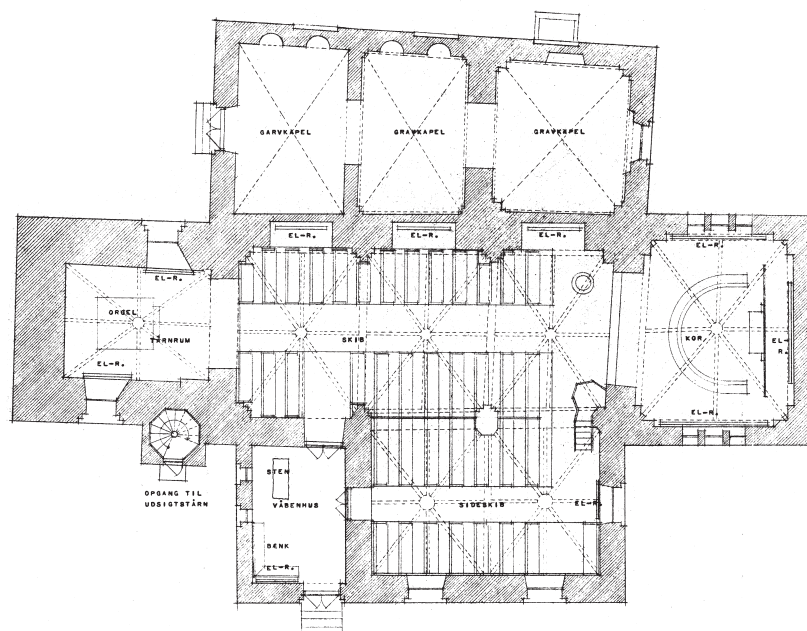
Fig. 110. Plan. 1:300. Målt og tegnet af Lars Mindedal 1978. – Plan.
