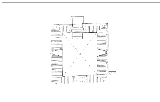
Fig. 109. Grundplan af gravkrypt. 1:300. Målt af Lars Mindedal 1978, suppleret og tegnet af Pia K. Lindholt 2019. Signaturforklaring s. 7. — Ground plan of burial crypt. Key on p. 7.
