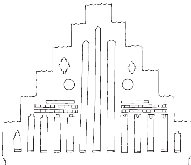
Fig. 71. Opstalt af nordkapellets trekantsgavl (s. 3030). 1:100. Målt og tegnet af Anders C. Christensen 2019. – Elevation of the pediment of the north chapel.
