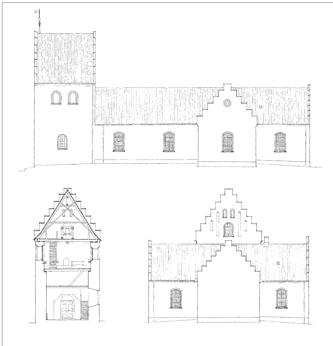
Fig. 14a-c. a. Opstalt af sydfacade. b. Tværnit gennem tårnet set mod øst. c. Opstalt af østfacade. 1:300. Målt og tegnet af Lars Mindedal 1986. — a. Elevation of the south facade. b. Section through tower looking east. c. Elevation of the east facade.
