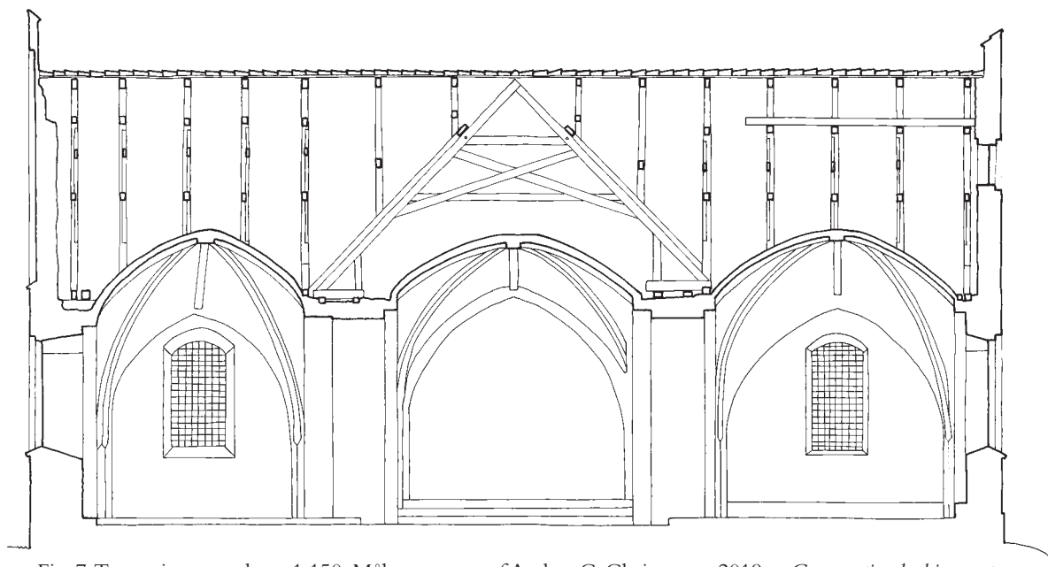
Fig. 7. Tværsnit set mod øst. 1:150. Målt og tegnet af Anders C. Christensen 2019. – Cross section looking east.
