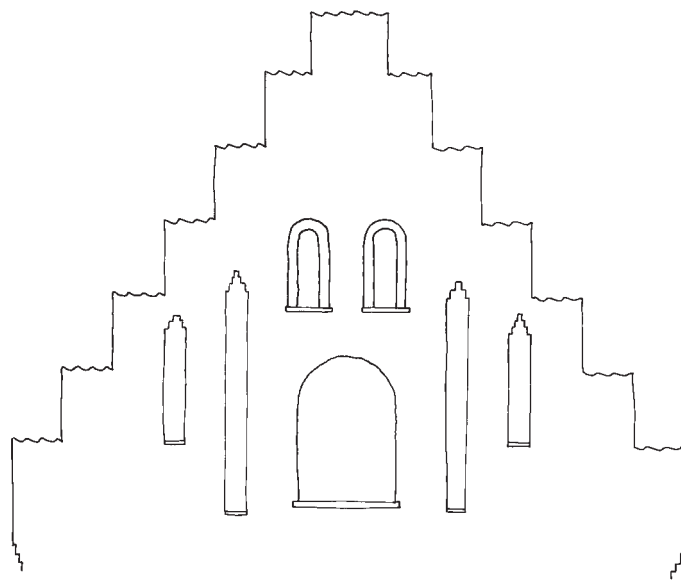
Fig. 72. Opstalt af tårnets østre gavltrekan (s. 3036). 1:100. Målt og tegnet af Anders C. Christensen 2019. – Elevation of the pediment of the tower.
