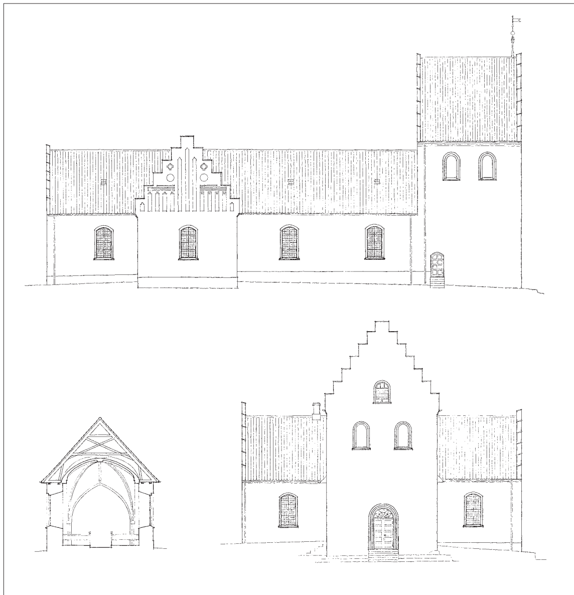
Fig. 14d-f. d. Opstalt af nordfacade. b. Tværsnit gennem skibet set mod vest. c. Opstalt af vestfacade. 1:300. Målt og tegnet af Lars Mindedal 1986. – a. Elevation of the north facade. b. Section through nave looking west. c. Elevation of the west facade.
