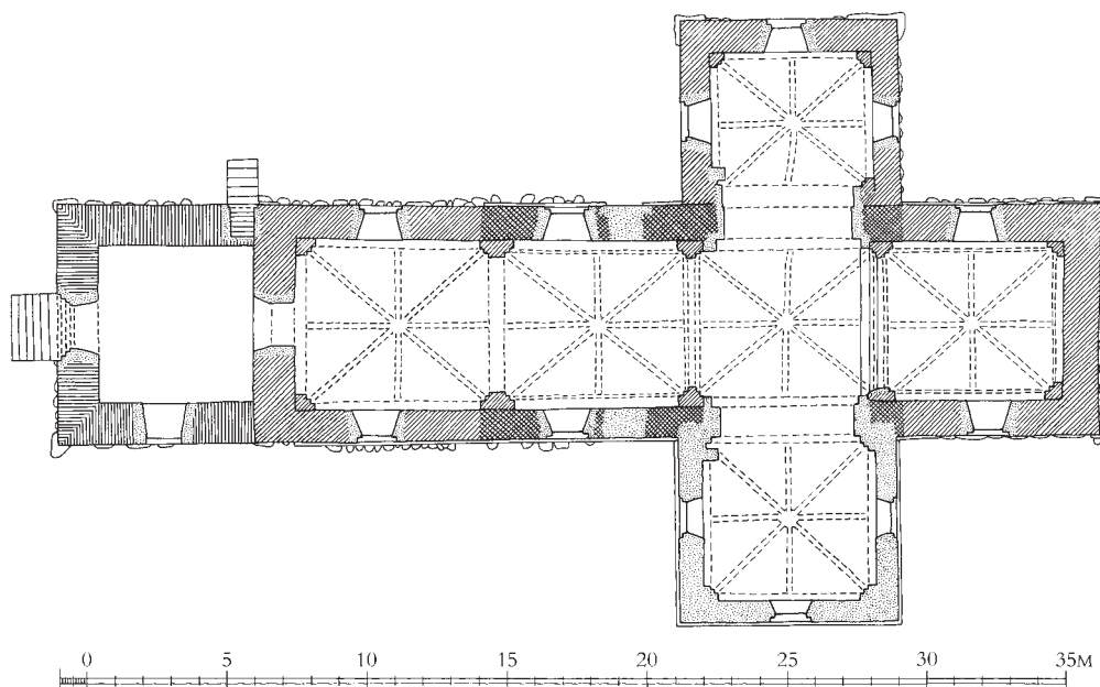
Fig. 8. Plan. 1:300. Målt af Lars Mindedal 1986, suppleret og tegnet af Anders C. Christensen 2020. Signaturforklaring s. 9. – Plan. Key on p. 17.
