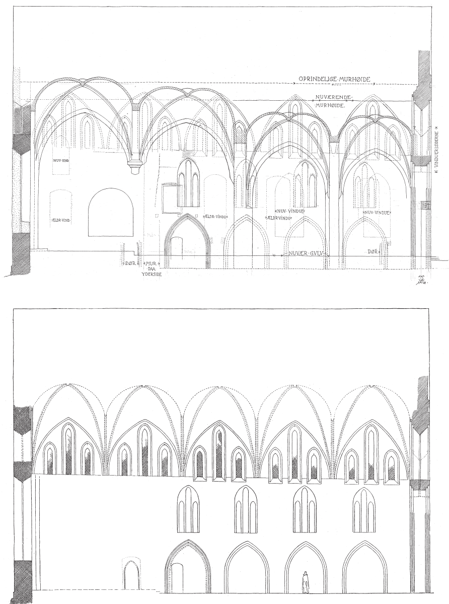
Fig. 176a-b. Længdesnit og rekonstruktion set mod syd. 1:300. Målt og tegnet af Ch. Christensen 1938. I NM. – Longitudinal section and reconstruction, looking south.
