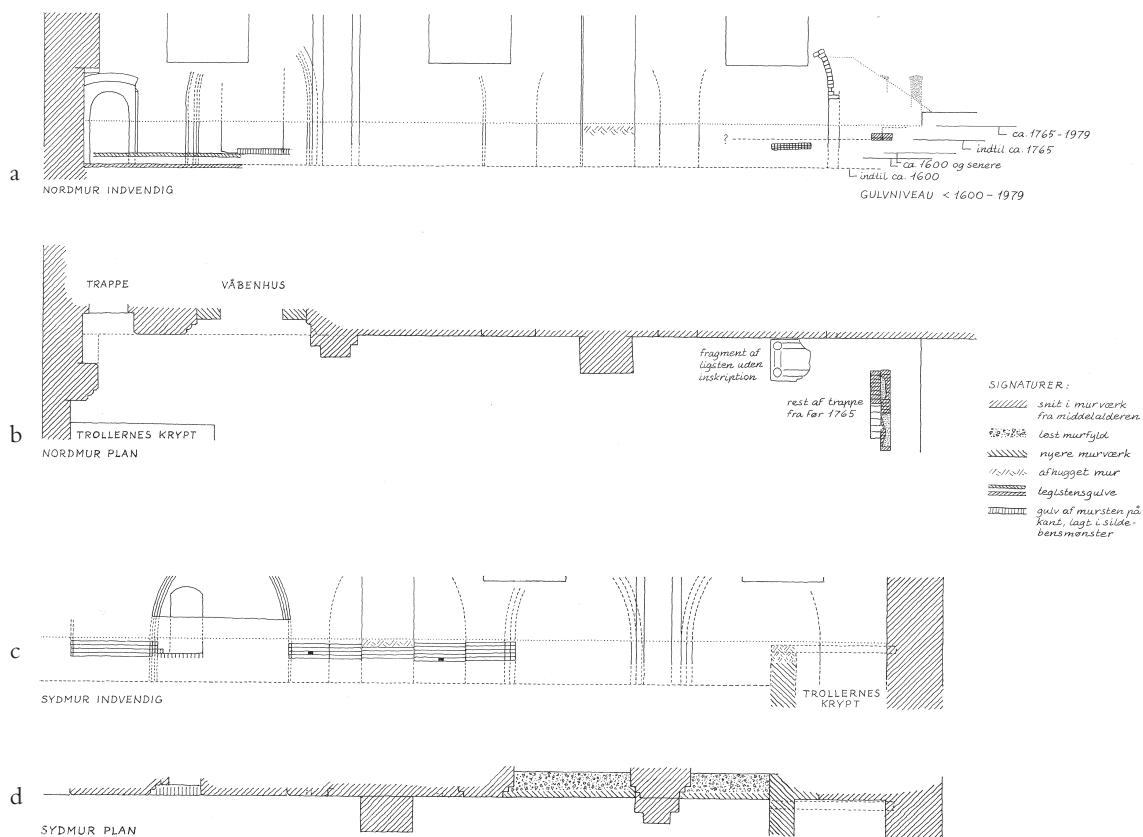
Fig. 88a-d. Opstalter og planer af skibet ved istandsættelsen 1988-89 (s. 3389). 1:200. a-b. Skibets nordside. c-d. Skibets sydside. Målt og tegnet af Jens Chr. Varming 1988-89. I Varmings Tegnestue. — Elevations and plans of the nave with the refurbishing of 1988-89. a-b. North side of the nave. c-d. South side of the nave.
