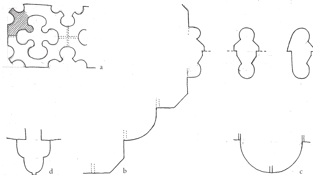
Fig. 179a-d. Formsten fra kirken. 1:10. a. Sten fra gesimsfrise (s. 3363). b. Profil af og stavværk i højkirkevindue i nord (s. 3365). c. Halvsøjle i nordre sideskib (s. 3354). d. Ribbesten i kirkens tre vestligste fag (s. 3375). Målt og tegnet af Ch. Christensen 1938. – Moulded bricks from the church. a. Bricks from the cornice frieze. b. Profile of and bar tracery in high church window in the north. c. Half-column in northern side aisle. d. Rib bricks in the three westernmost bays of the church.
