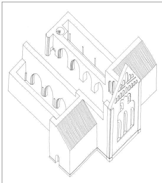
Fig. 39. Rekonstruktion af kirkens 2. byggefase, o. 1275, set fra sydøst. 1:600. Tegnet af Pia K. Lindholt 2022. – Reconstruction of the second construction phase of the church, c. 1275, seen from the south east.
