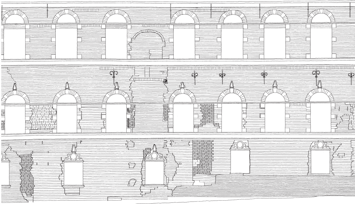
Fig. 36. Opstalt af østfløjens østfacade set fra øst (s. 3345). Middelalderligt murværk har skråravering. 1:150. I Varmings Tegnestue. – Elevation of the east facade of the east wing seen from the east.
