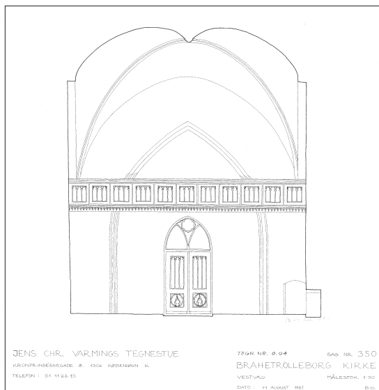
Fig. 79. Kirkens vestvæg med ÷pulpitur (s. 3426) set mod vest. 1:200. Målt og tegnet af Birte Skov 1987. I Varmings Tegnestue. — The west wall of the church with ÷gallery, looking west.
