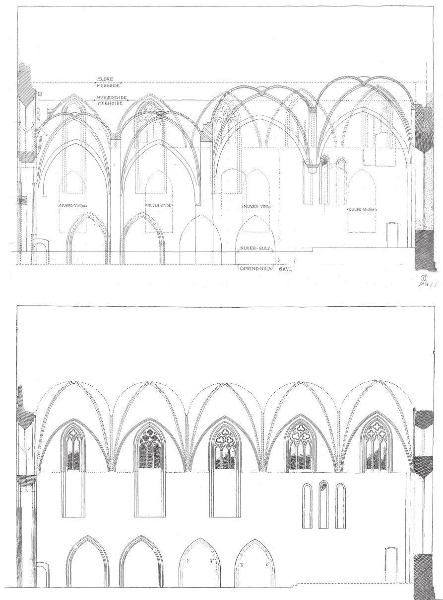
Fig. 176c-d. Længdesnit og rekonstruktion set mod nord. 1:300. Målt og tegnet af Ch. Christensen 1938. I NM. – Longitudinal section and reconstruction, looking north.
