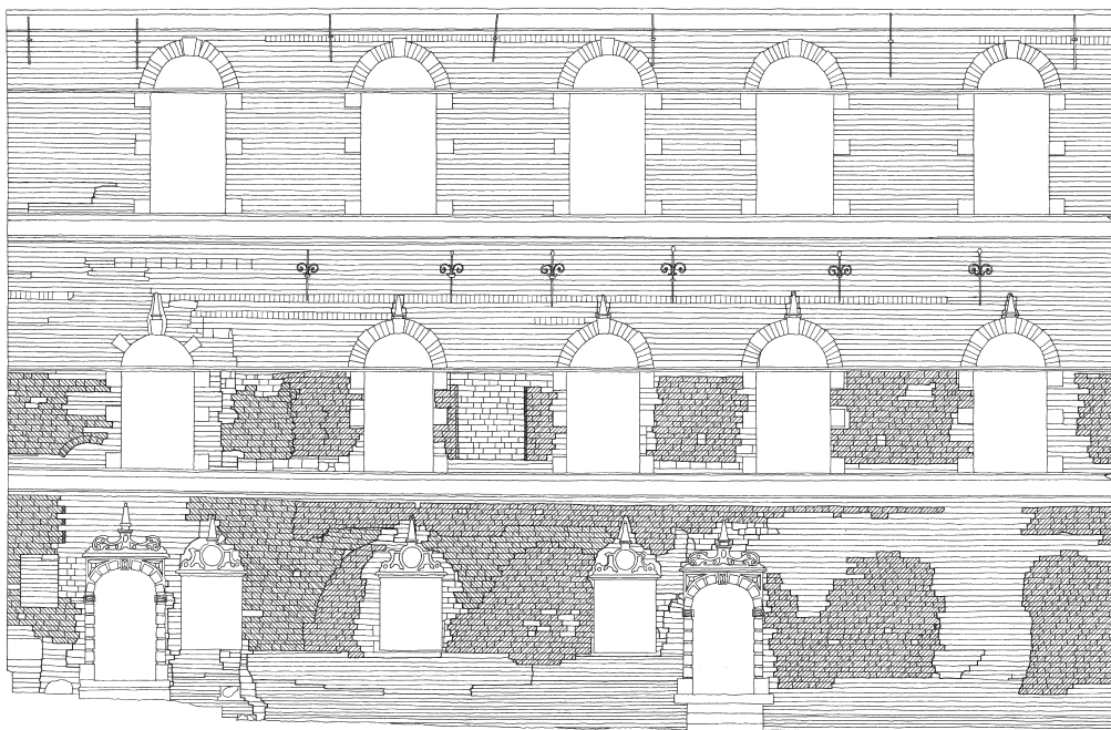
Fig. 44. Opstalt af østfløjens vestfacade set fra vest (s. 3323). Middelalderligt murværk har skråkrave-ring. 1:150. I Varmings Tegnestue. – Elevation of the west facade of the east wing seen from the west.
