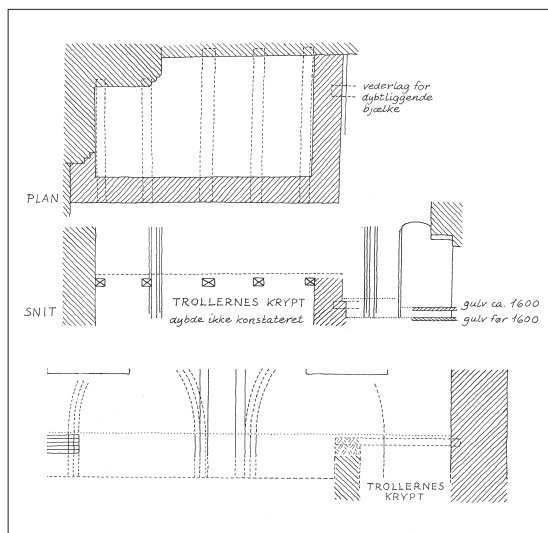
Fig. 78a-c. Den trolleske krypt (s. 3381). 1:200. a. Plan (vest opad). b. Snit set mod vest. c. Snit set mod syd. Målt og tegnet af Jens Chr. Varming 1988-89. I Varmings Tegnestue. — The Trolle crypt. a. Plan. b. Section looking west. c. Section looking south.
