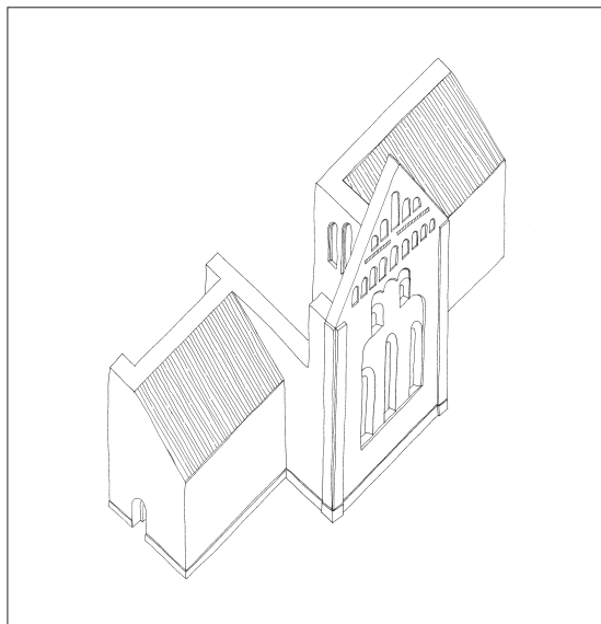
Fig. 33. Rekonstruktion af kirkens 1. byggefase, 1225-50, set fra sydøst. 1:600. Tegnet af Pia K. Lindholt 2022. – Reconstruction of the first construction phase of the church, 1225-50, seen from the south east.
