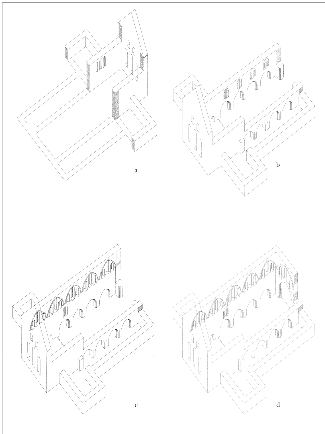
Fig. 181a-d. Rekonstruktion af kirkens byggefaser. 1:600. Tolket og tegnet af Ebbe Hædersdal 1990. I privateje og efter Hædersdal 1990. – Reconstruction of the construction phases of the church.
