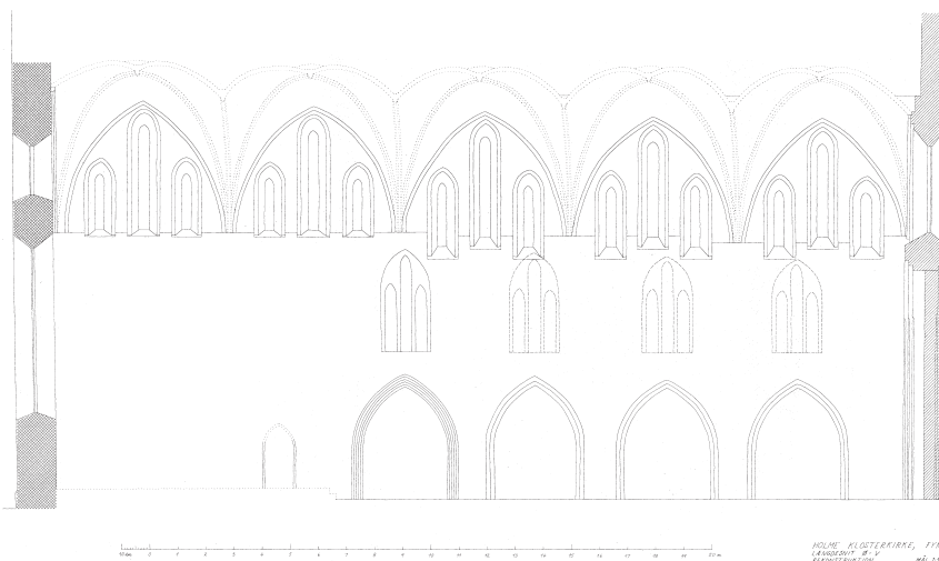
Fig. 30a-e. a. Længdesnit set mod nord. b. Rekonstruktion af længdesnit set mod nord. c. Længdesnit af nuværende forhold set mod nord. d. Længdesnit set mod syd. e. Rekonstruktion af længdesnit set mod syd. 1:300. Målt og tegnet af Ebbe Hædersdal 1990 efter Ch. Christensen 1938. I privateje. — a. Longitudinal section, looking north. b. Reconstruction of longitudinal section, looking north. c. Longitudinal section in present state, looking north. d. Longitudinal section, looking south. e. Reconstruction of longitudinal section, looking south.
