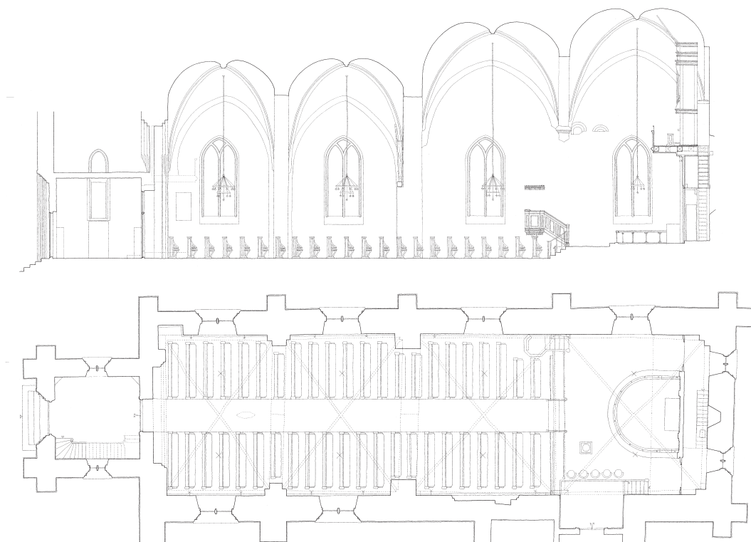
Fig. 186a-b. a. Længdesnit. Målt og tegnet af Jens Chr. Varming 1987 og 2002. b. Grundplan. Målt og tegnet af Birte Skov 1987. 1:300. I Varmings Tegnestue. – a. Longitudinal section. b. Ground plan.
