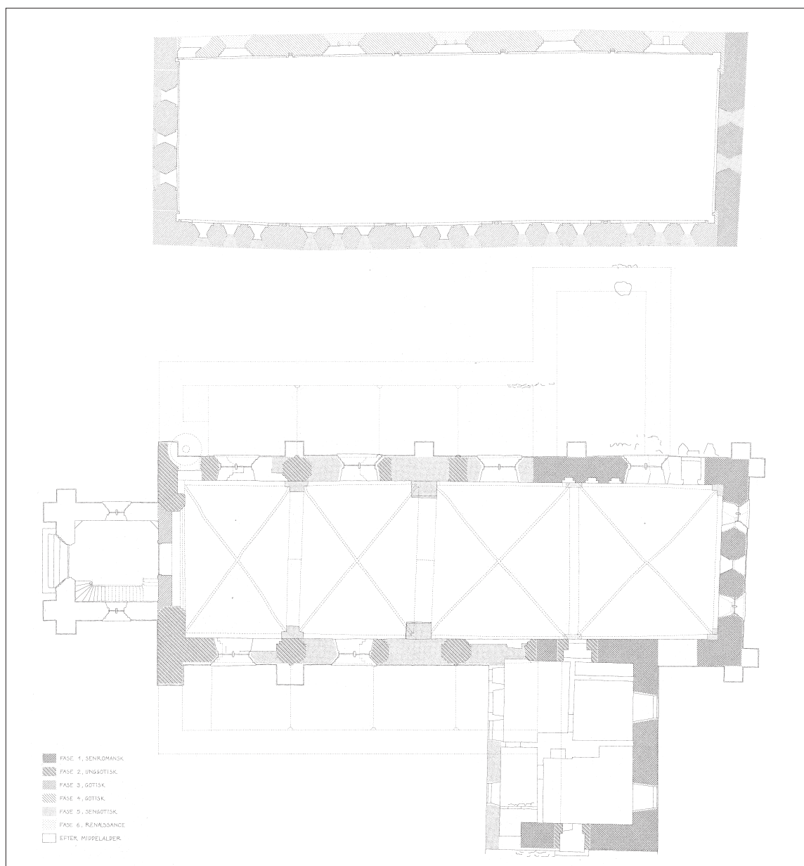
Fig. 180a-b. a. Højkirkens vinduesstokværk, delvist rekonstrueret. Målt og tegnet af Ebbe Hædersdal 1990. b. Grundplan med forsvundne bygningsdele. Målt og tegnet af Ebbe Hædersdal 1990 efter forlæg af Ch. Christensen 1938 samt Birte Skov og Jens Chr. Varming 1989. 1:300. I privateje. – a. Window floor of high church, partly reconstructed. b. Ground plan with missing parts of the building.
