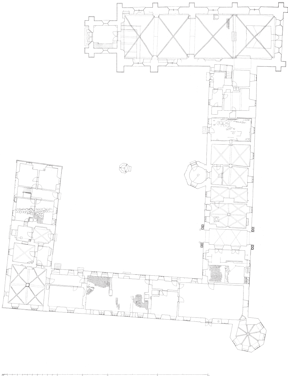
Fig. 32. Oversigtsplan af klostret. 1:400. Tegnet af Jens Chr. Varming o. 1990. I Varmings Tegnestue. — General plan of the monastery.
