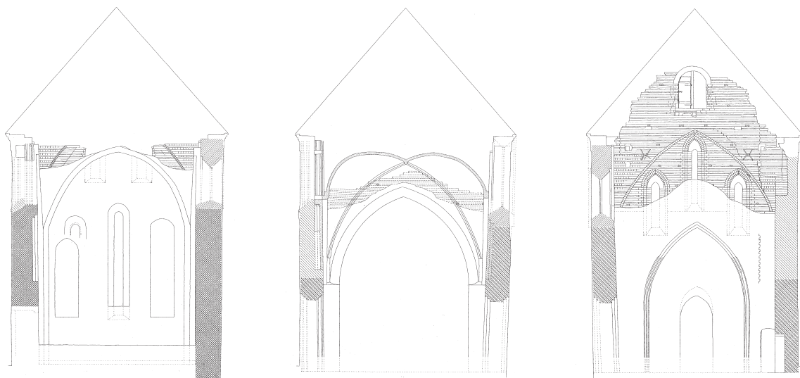
Fig. 31a-c. a. Tværsnit gennem koret set mod øst. b. Tværsnit gennem tredje hvælvfag set mod øst. c. Tværsnit gennem fjerde hvælvfag set mod vest. 1:300. Målt og tegnet af Ebbe Hædersdal 1990 efter Ch. Christensen 1938. Efter Hædersdal 1990. – a. Cross-section through the chancel, looking east. b. Cross-section through the third vault bay, looking east. c. Cross-section through the fourth vault bay, looking west.
