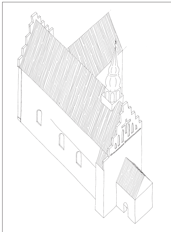
Fig. 80. Rekonstruktion af kirken efter tilføjelse af våbenhus ved vestgavlen 1817 (s. 3382). 1:600. Set fra nordvest. Tegnet af Pia K. Lindholt 2022. – Reconstruction of the church after the addition of a porch at the west gable in 1817. Seen from the north west.
