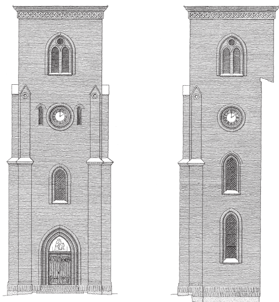
Fig. 85a-b. Opstalter af tårnets vest- og sydfacader (s. 3388). 1:300. Målt og tegnet af Jens Chr. Varming 1995. I Varmings Tegnestue. – Elevations of the west and south facades of the tower.
