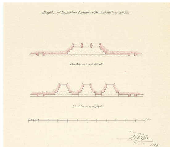
Fig. 22. Plan af højirkens nord- og sydvinduer. 1: 150. Tegnet af J. B. Løffler 1886. I NM. – Plan of the north and south windows of the high church.
