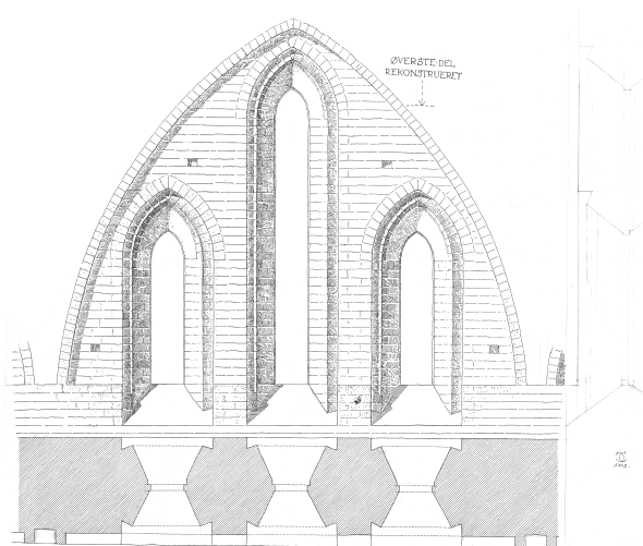
Fig. 178a. Rekonstruktion og plan af et fag af de søndre højkirkevinduer (s. 3357). 1:100. Målt og tegnet af Ch. Christensen 1938. I NM. – Reconstruction and plan of a bay of the southern high church windows.
