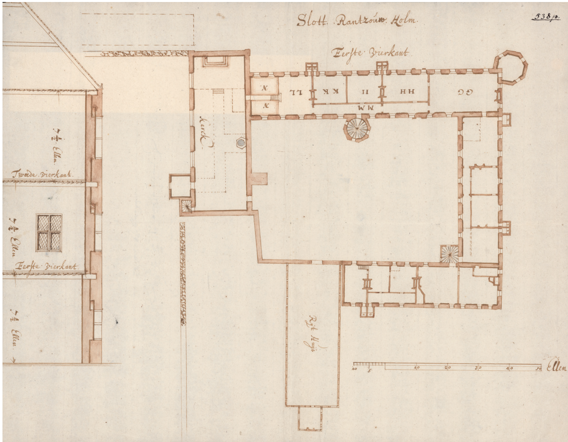
Fig. 21a-b. Rantzausholm o. 1660. a. Plan af herregården. Øst opad. b. Snit gennem østfløjen. I NM. – Rantzausholm c. 1660. a. Plan of manor house, east upward. b. Section through the east wing.
