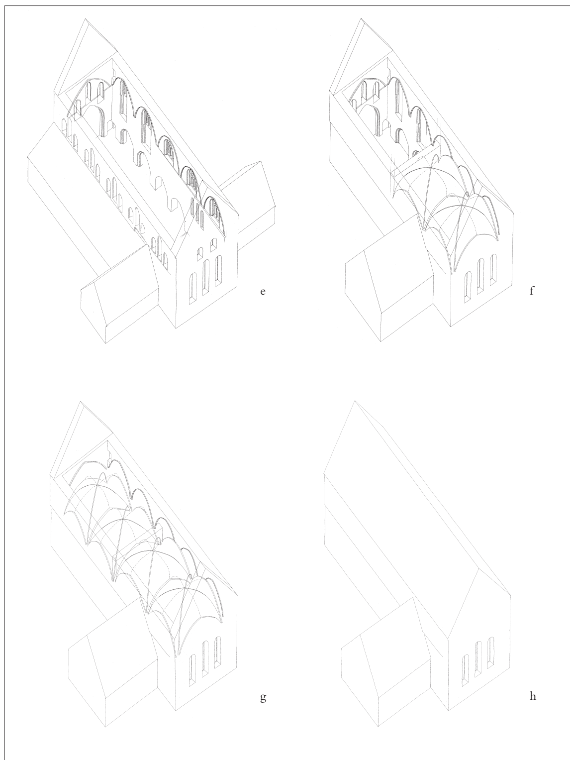
Fig. 181e-h. Rekonstruktion af kirkens byggefaser. 1:600. Tolket og tegnet af Ebbe Hædersdal 1990. I privateje og efter Hædersdal 1990. – Reconstruction of the construction phases of the church.
