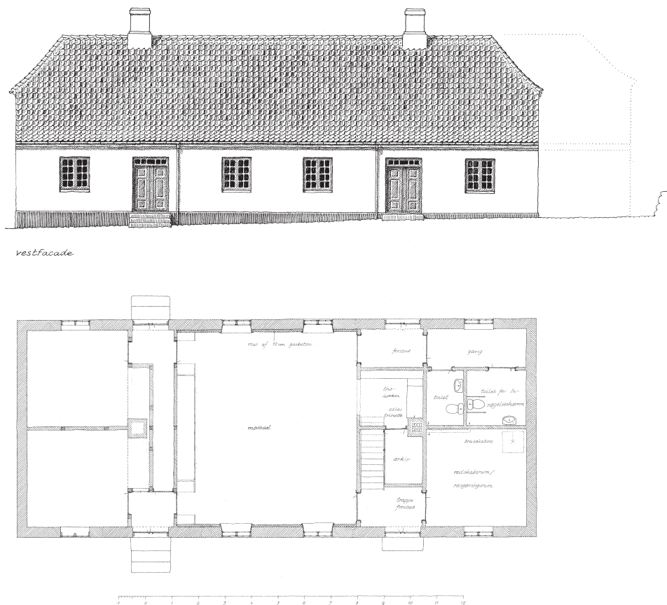
Fig. 7-8. Forslag til ombygning af hospitalet (s. 3319). 1:200. I Varmings Tegnestue. 7. Vestfacade. Tegnet af Jens Chr. Varming 1981. 8. Plan. Tegnet af L. Topsøe-Jensen 1982-83. – Proposal for the rebuilding of the hospital. 7. West facade. 8. Plan.
