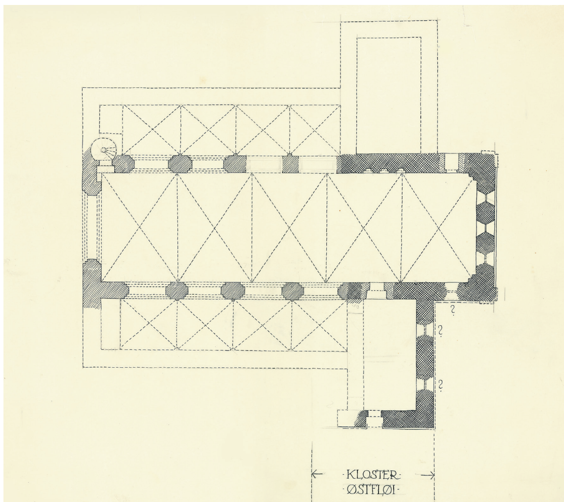
Fig. 175a–c. Rekonstruktion af kirkens tre stokværk. a. Kirkens nedre stokværk. b. Kirkens blændingsstokværk. c. Højkirkens vinduesstokværk. 1:300. Målt og tegnet af Ch. Christensen 1938. I NM. – Reconstructions. a. The lower floor of the church. b. The recessed floor of the church. c. The window floor of the high church.
