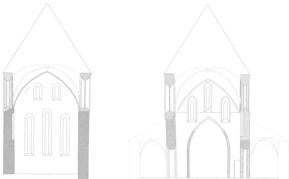
Fig. 31d-e. d. Rekonstrueret tværsnit gennem koret set mod øst. e. Rekonstrueret tværsnit gennem kirken set mod vest. 1:300. Målt og tegnet af Ebbe Hædersdal 1990 efter Ch. Christensen 1938. Efter Hædersdal 1990. – d. Reconstructed cross-section through the chancel, looking east. e. Reconstructed cross-section through the church, looking west.
