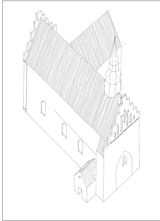
Fig. 77. Rekonstruktion af kirken efter tilføjelse af våbenhus på nordsiden i begyndelsen af 1600-tallet (s. 3381). 1:600. Set fra nordvest. Tegnet af Pia K. Lindholt 2022. – Reconstruction of the church after the addition of a porch on the north side at the beginning of the 1600s. Seen from the north west.
