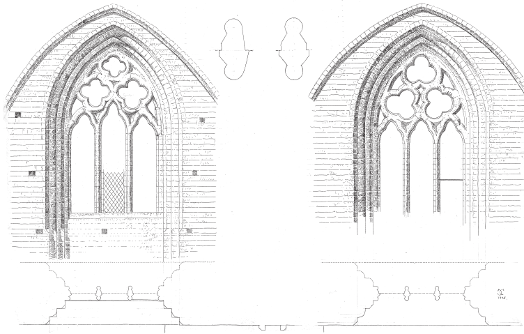
Fig. 178b. Rekonstruktion og plan af det nordre højkirkevindue i fjerde og tredje fag (s. 3365). 1:100. Målt og tegnet af Ch. Christensen 1938. I NM. – Reconstruction and plan of the northern high church window in the fourth and the third bay.
