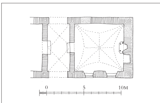
Fig. 3. Grundplan. 1:300. Målt og tegnet af Pia K. Lindholt 2022. Signaturforklaring s. 9. – Ground plan. Key on p. 17.
