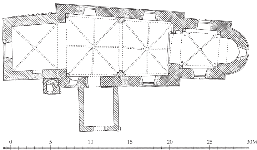
Fig. 10. Grundplan. 1:300. Målt af Axel Jacobsen 1958, suppleret og tegnet af Pia K. Lindholt 2024. Signaturforklaring s. 9. – Plan. Key on p. 17.
