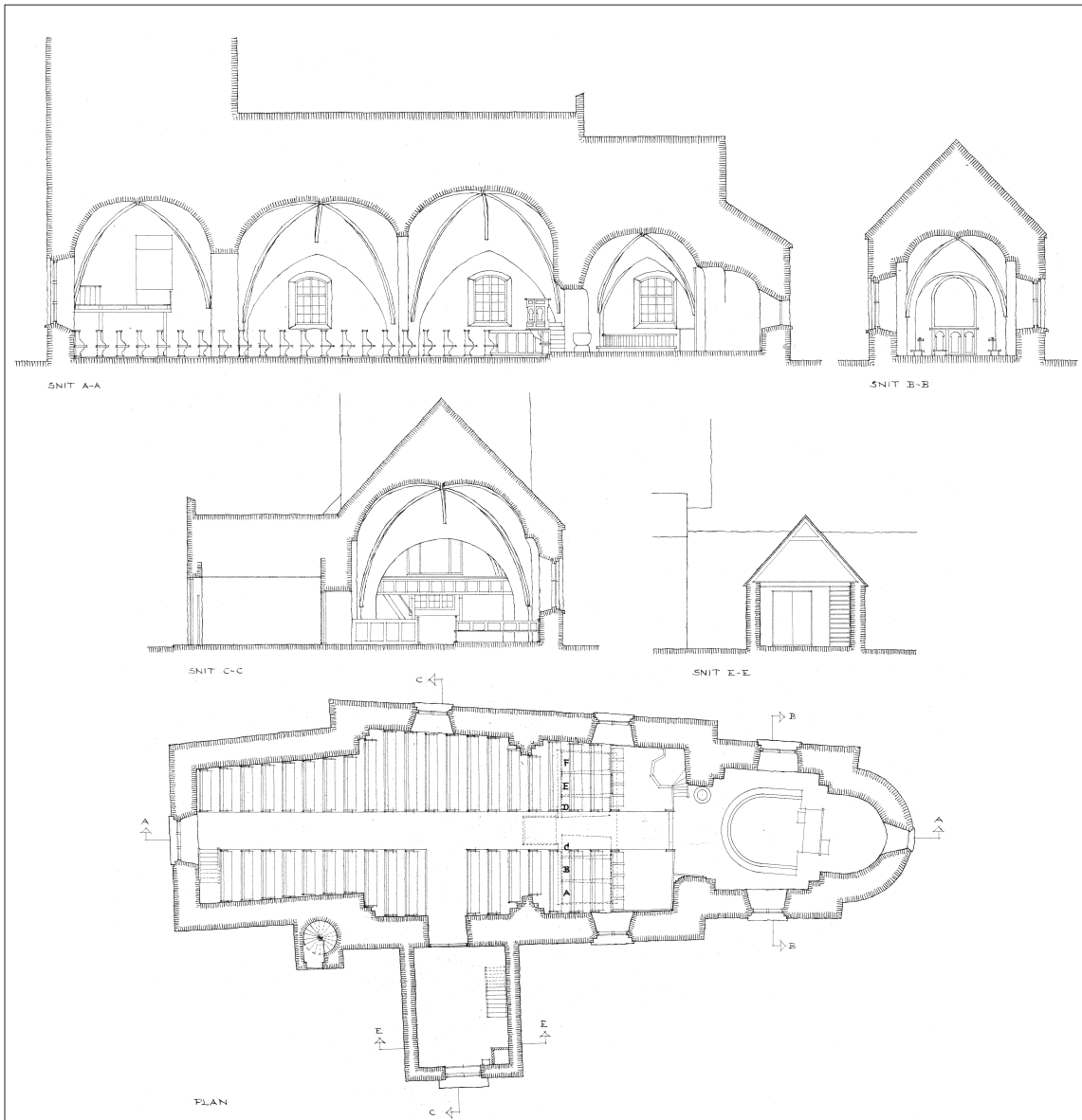
Fig. 20a-e. Opmåling af kirken med forslag til ændringer 1961. 1:300. a. Længdesnit set mod nord. b. Tværsnit gennem kor set mod øst. c. Tværsnit gennem skibets andet fag og våbenhus set mod vest. d. Tværsnit gennem våbenhus set mod nord. e. Plan. Målt og tegnet af Axel Jacobsen 1961. I NM. – Scale drawing of the church with proposals for changes, 1961. a. Longitudinal section looking north. b. Cross-section through the chancel looking east. c. Cross-section through the porch and the second bay of the nave looking west. d. Cross-section through the porch looking north. e. Plan.
