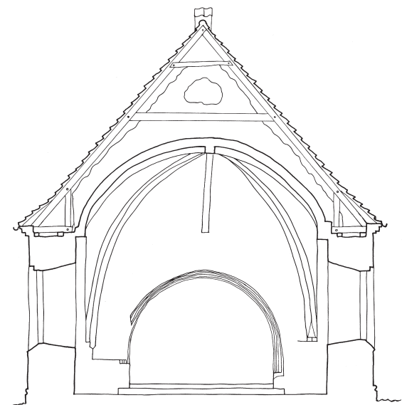
Fig. 9. Tværsnit. 1:150. Målt og tegnet af Pia K. Lindholt 2024. – Cross-section.
