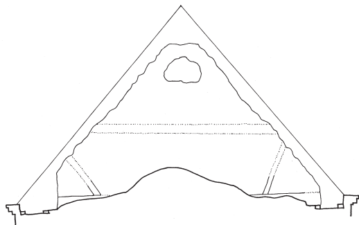
Fig. 95. Opmåling af skibets østgavl med aftryk af det romanske tagværk (s. 4133). Nederst aftryk af bindbjælke og skråstivere og øverst markering af hanebånd. 1:150. Målt af Cæcilie H. M. Thomsen og Pia K. Lindholt, tegnet af sidstnævnte 2024. – Scale drawing of the nave's eastern gable with impressions from the Romanesque roofing. Below are the marks of a tie beam and struts and above is the mark of the collar beam.
