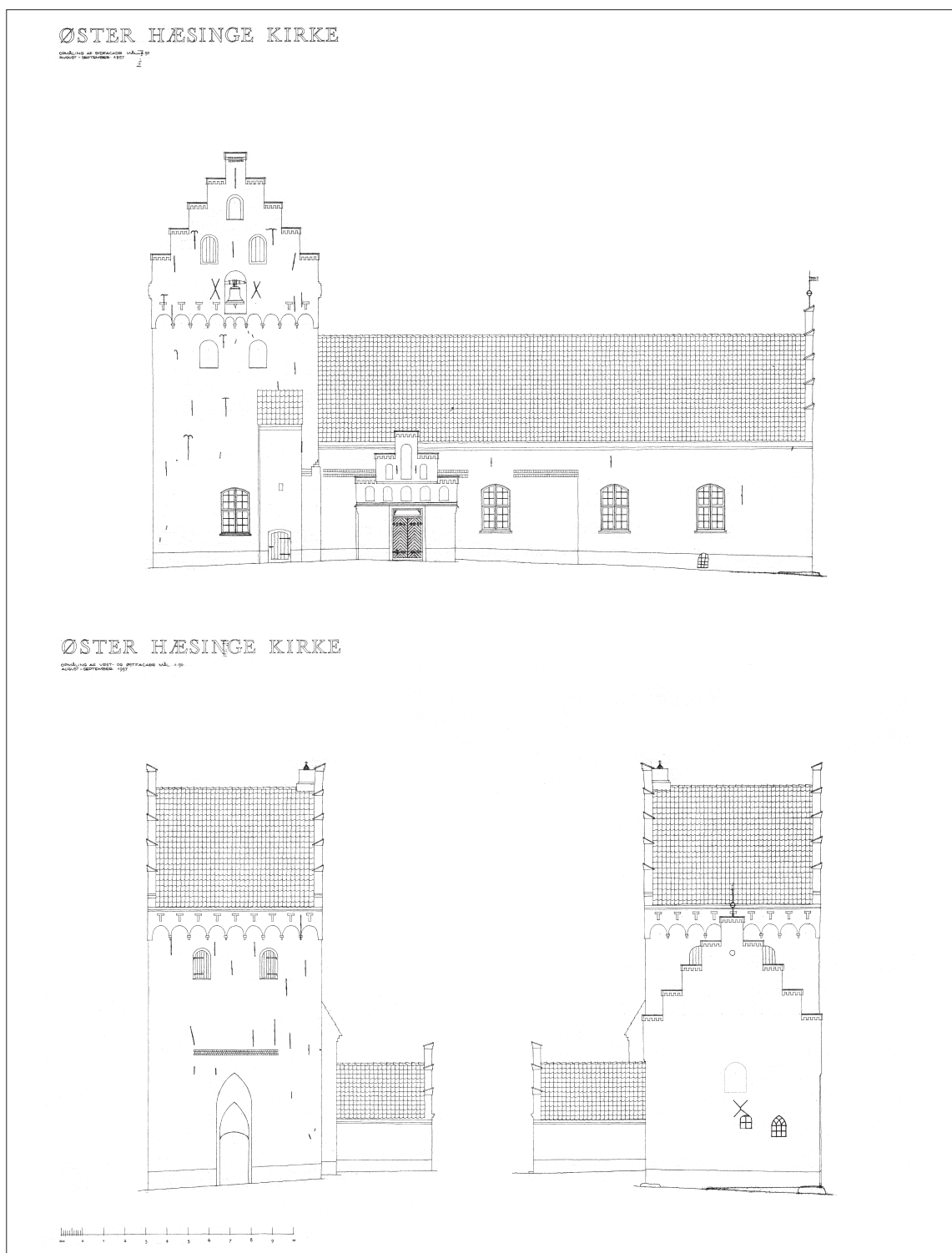
Fig. 20e-g. Opmåling inden istandsættelsen 1964-65 (s. 4213). 1:300. Facadeopstalter. e. Sydfacade. f. Vestfacade. g. Østfacade. Målt og tegnet af Lars Mindedal Rasmussen og Sven Wilhelmsen 1957. I NM. — Scale drawing before the refurbishing in 1964-65. Elevations of facades. e. South facade. f. West facade. g. East facade.
