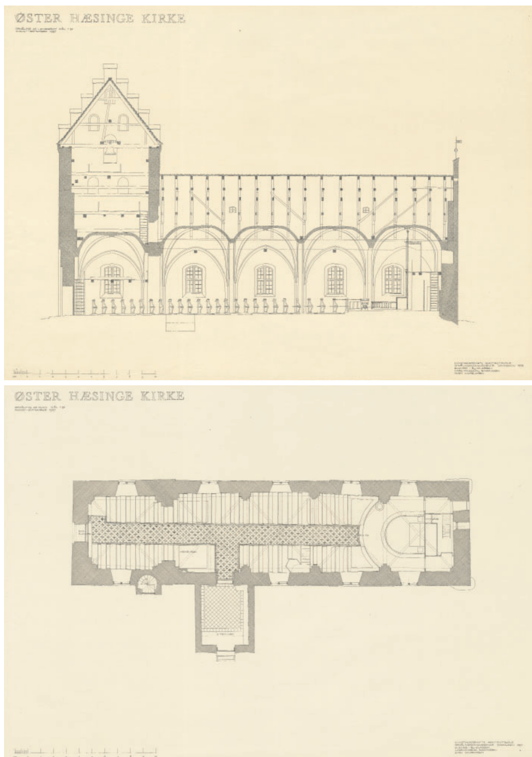
Fig. 20a-b. Opmåling inden istandsættelsen 1964-65 (s. 4213). 1:300. a. Længdesnit set mod nord. b. Plan. Målt og tegnet af Lars Mindedal Rasmussen og Sven Wilhelmsen 1957. I KB. Kunstbiblioteket. — Scale drawing before the refurbishing in 1964-65. a. Longitudinal section looking north. b. Plan.
