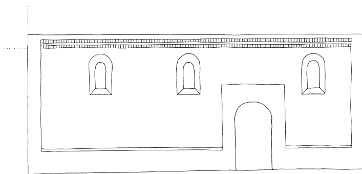
Fig. 100. Rekonstruktion af skibets romanske nordfacade (s. 4199). 1:150. Målt af Lars Mindedal Rasmussen og Sven Wilhelmssen 1957, suppleret og tegnet af Pia K. Lindholt 2024. – Reconstruction of the nave's Romanesque north facade.
