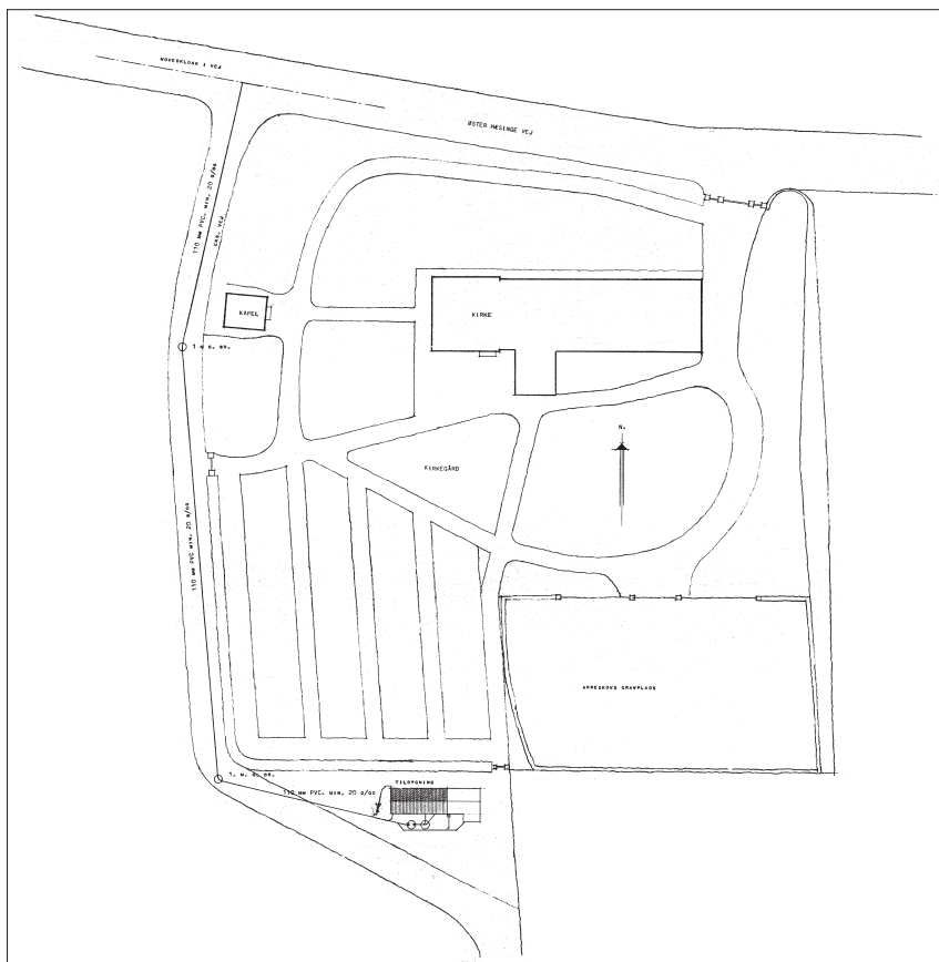
Fig. 4. Situationsplan. 1:1000. Målt af Lars Mindedals Tegnesteue 1986. – Situation plan.
