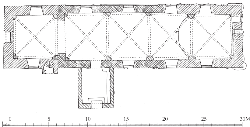
Fig. 11. Grundplan. 1:300. Målt af Lars Mindedal Rasmussen og Sven Wilhelmsen 1957, suppleret og tegnet af Pia K. Lindholt 2024. Signaturforklaring s. 9. – Ground plan. Key on p. 17.
