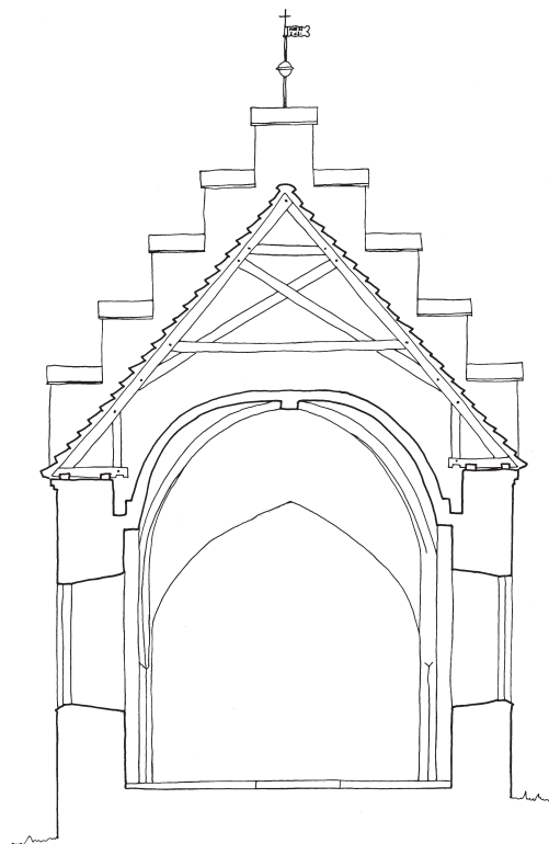
Fig. 10. Tværnsnit. 1:150. Målt af Lars Mindedal Rasmussen og Sven Wilhelmsen 1957, suppleret og tegnet af Pia K. Lindholt 2024. – Cross-section.
