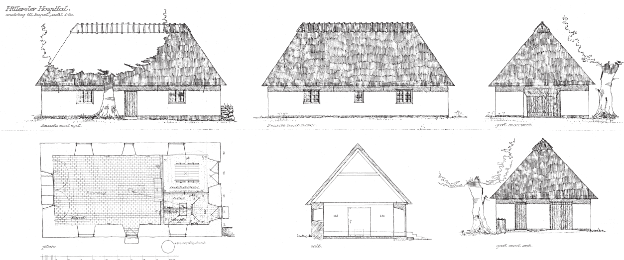
Fig. 92. Forslag til ombygning af hospitalet (s. 4284). a. Grundplan. b. Tværsnit set mod syd. c. Opstalter af facader. 1:300. Målt og tegnet af Ejnar Mindedal Rasmussen 1957. I NM. – Proposal for the rebuilding of the hospital. a. Ground plan. b. Cross-section looking south. c. Elevations of facades.
