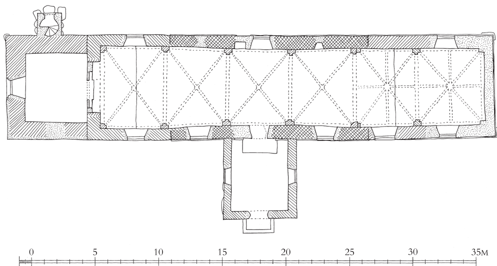
Fig. 7. Grundplan. 1:300. Målt af Ejnar Mindedal Rasmussen 1939, suppleret og tegnet af Pia K. Lindholt 2024. Signaturforklaring s. 9. – Ground plan. Key on p. 17.
