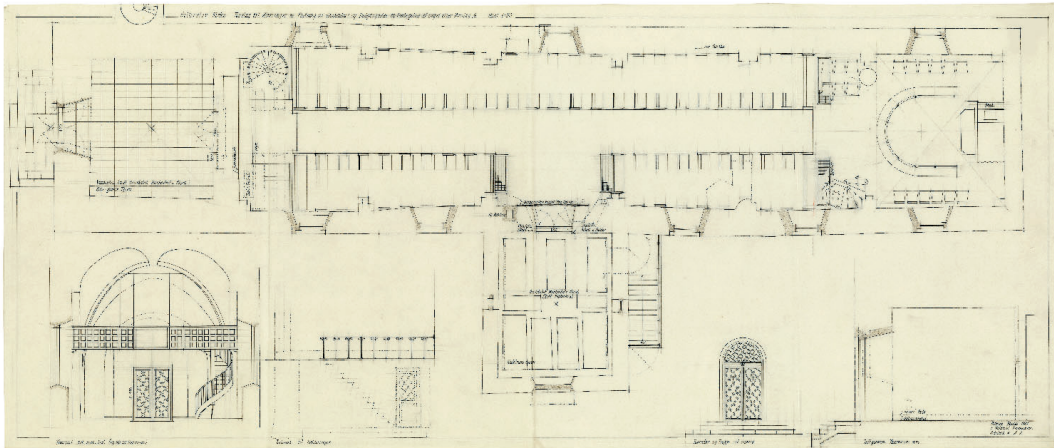
Fig. 97. Forslag til ændring af adgangsforhold til kirken (s. 4297). a. Grundplan. b. Tværnsnit gennem vestforlængelsen set mod vest. c. Længdesnit gennem tårnrum. d. Vestdør. e. Opstalt af trappe til fyrrum under våbenhuset. 1:300. Målt og tegnet af Ejnar Mindedal Rasmussen 1941. I NM. – Proposal for changing the entrances to the church. a. Ground plan. b. Cross-section through the western extension looking west. c. Longitudinal section through the tower interior. d. West door. e. Elevation of the staircase to the boiler room below the porch.
