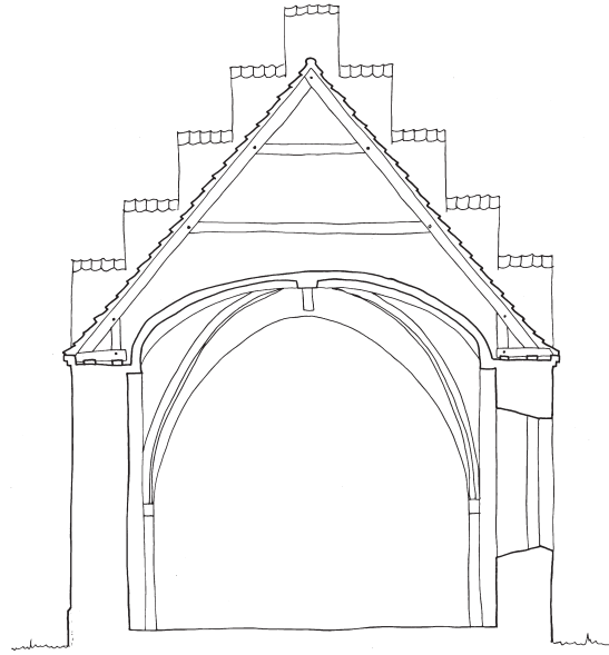
Fig. 8. Tværsnit. 1:150. Målt af Lars Mindedal 1981, suppleret og tegnet af Pia K. Lindholt 2024. – Cross-section.
