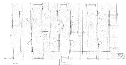
Fig. 93. Grundplan af hospitalet med indretning fra 1769 (s. 4284). 1:300. Målt og tegnet af Ejnar Mindedal Rasmussen o. 1957. I NM. – Ground plan of the hospital.
