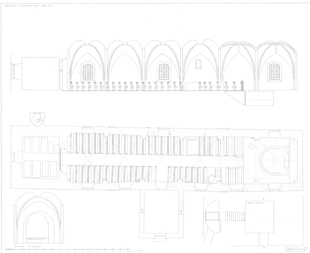
Fig. 20a-e. Opmåling inden istandsættelsen 1942-43 (s. 4297). a. Grundplan. b. Længdesnit. c. Tværnsnit gennem vestforlængelsen set mod vest. d. Tværnsnit gennem \ddagger krypt under koret. e. Grundplan af \ddagger krypt under koret. 1:300. Målt og tegnet af Ejnar Mindedal Rasmussen 1939. I NM. – Scale drawing before the refurbishing of 1942-43. a. Ground plan. b. Longitudinal section. c. Cross-section through the western extension looking west. d. Cross-section through the \ddagger crypt below the chancel. e. Ground plan of the \ddagger crypt below the chancel.
