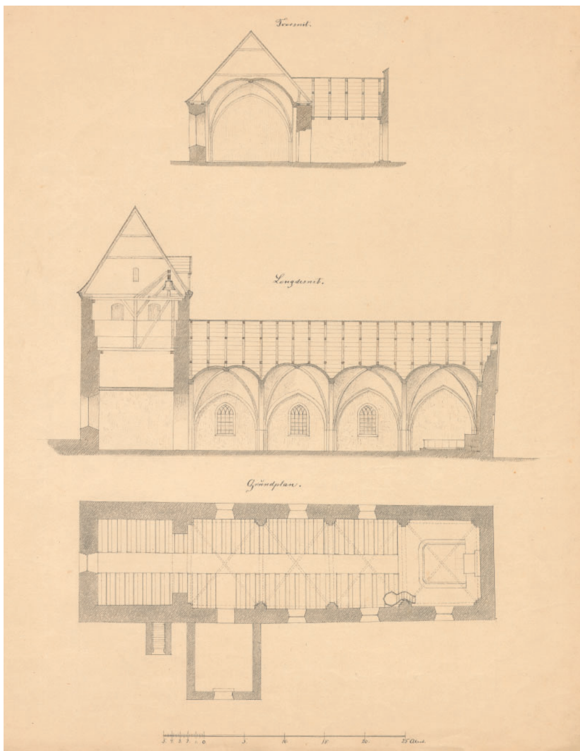
Fig. 12e-g. Opmåling af kirken o. 1890. 1:300. e. Tværsnit gennem fjerde fag og våbenhus set mod øst. f. Længdesnit set mod nord. g. Grundplan. Målt og tegnet af J. Vilh. Petersen o. 1890. I KB. Danmarks Kunstbibliotek. — Scale drawing of the church, c. 1890. e. Cross-section through the fourth bay and the porch looking east. f. Longitudinal section looking north. g. Ground plan.
