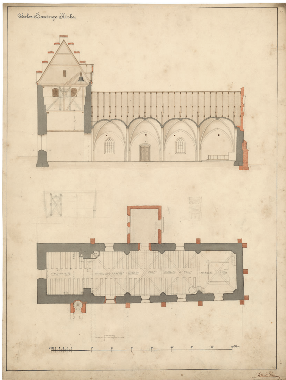
Fig. 13a-b. Opmåling af kirken med forslag til ændringer o. 1890. 1:300. a. Længdesnit set mod nord. b. Grundplan. Målt og tegnet af J. Vilh. Petersen o. 1890. I NM. — Scale drawing of the church with proposed changes, c. 1890. a. Longitudinal section looking north. b. Ground plan.
