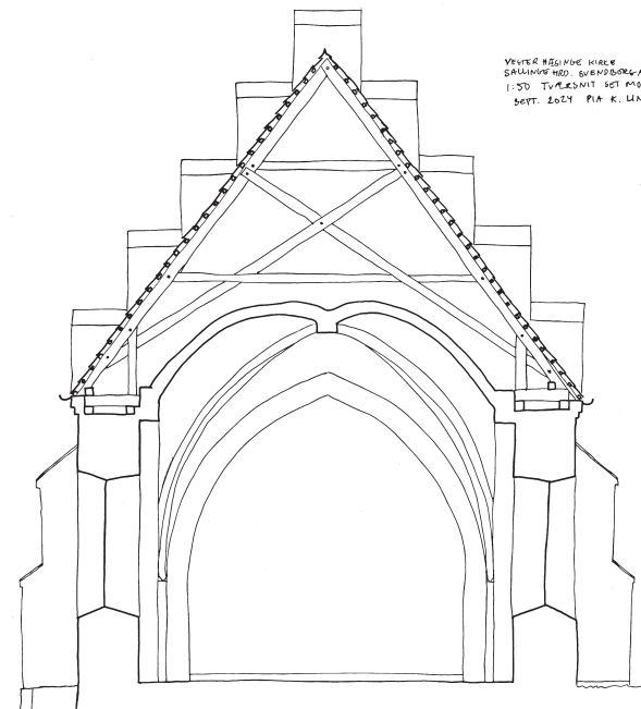
Fig. 9. Tværsnit. 1:150. Målt og tegnet af Pia K. Lindholt 2024. - Cross-section.
