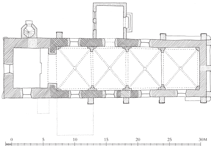
Fig. 8. Grundplan. 1:300. Målt af Krogh Madsens Arkitekttegnestue 2009, suppleret og tegnet af Pia K. Lindholt 2024. Signaturforklaring s. 9. - Ground plan. Key on p. 17.
