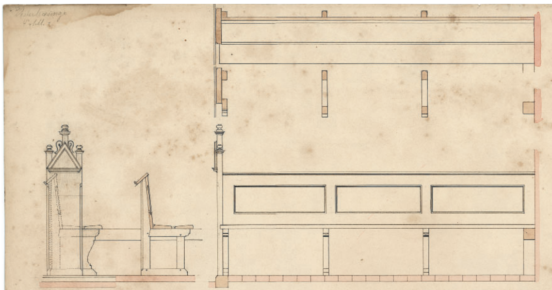
Fig. 39. Stolestader (s. 4390), tegnet af J. Vilh. Petersen 1892. I NM. – Current pews.
