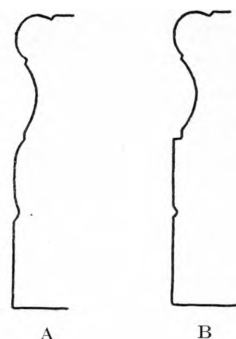
Fig. 5. Romanske Sokkelsten. 1:10. Maalt af C. G. Schultz 1937 (S. 30).
