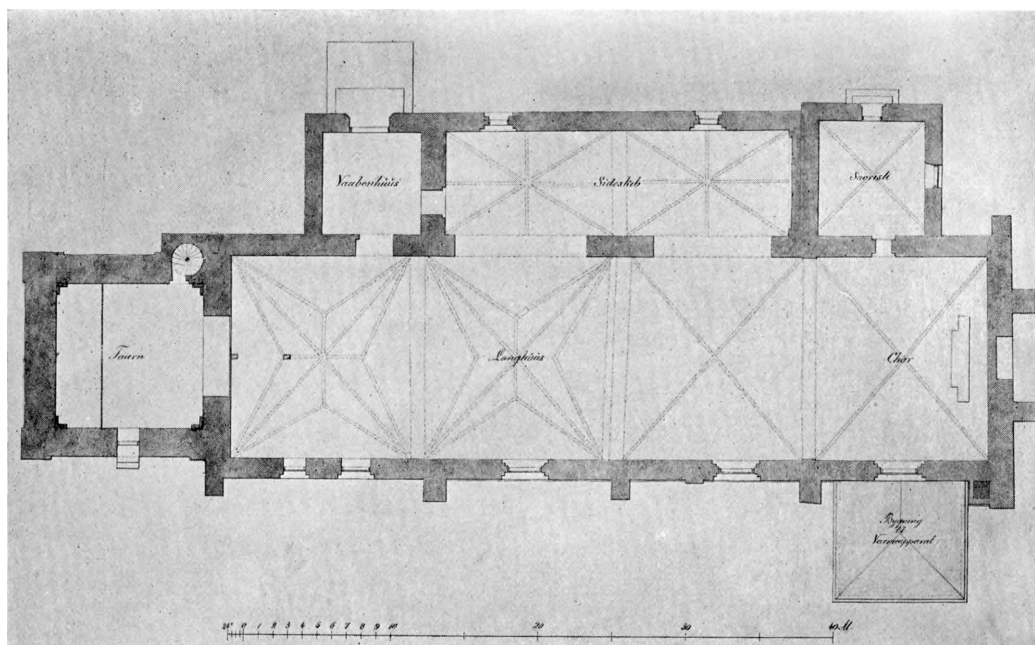
Fig. 2. Nykøbing. Den 1890 nedrevne Kirke. Plan. 1:300. Maalt af F. Uldall 1884.
