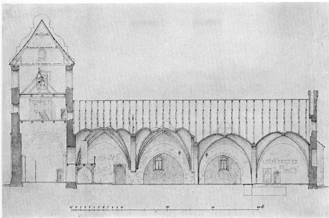
Fig. 3. Nykøbing. Den 1890 nedrevne Kirke. Snit, set mod Nord. 1:300. Maalt af F. Uldall 1884.
