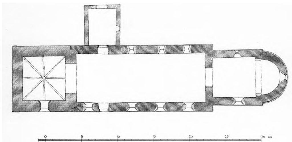
Fig. 2. Plan. 1:300. Maalt af C. G. Schultz 1936.
