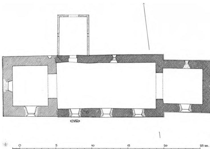
Fig. 2. Vester-Torup. Plan 1:300. Maalt af C. G. Schultz 1936.
