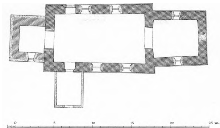
Fig. 2. Arup. Plan. 1:300. Maalt af C. G. Schultz 1936.
