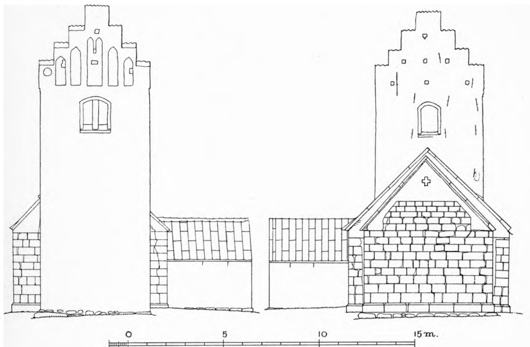
Fig. 3. Arup. Opstalt. 1:200. Set fra Vest og fra Øst, maalt af Gudmund Holme 1924.
