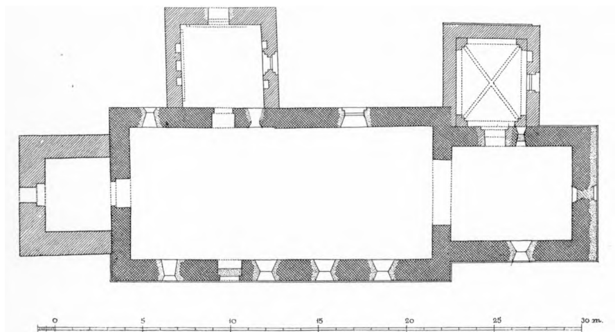
Fig. 2. Nors. Plan. 1 : 300. Maalt af C. G. Schultz 1936.
