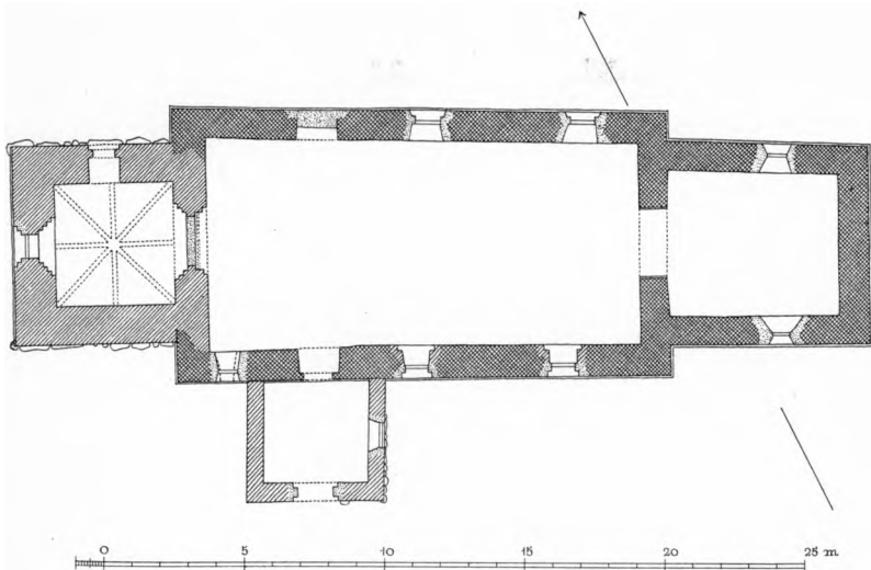
Fig. 2. Hunstrup. Plan. 1:300. Maalt af C. G. Schultz 1936.
