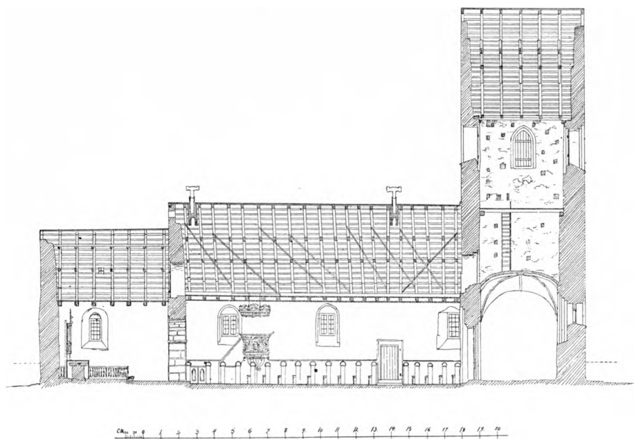
Fig. 3. Hunstrup. Længdesnit, set mod Syd. 1:300. Maalt af Hother Paludan 1917.
