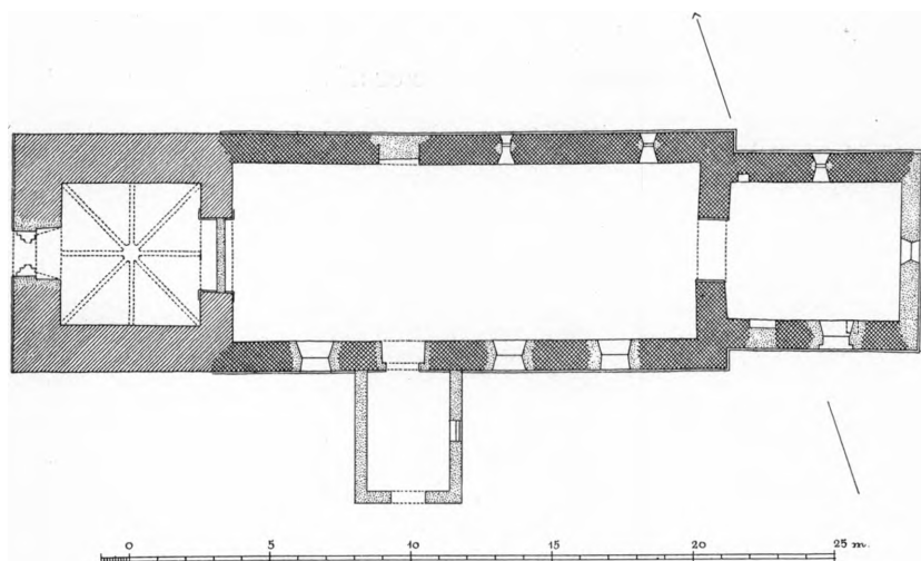
Fig. 2. Østerild. Plan. 1:300. Maalt af C. G. Schultz 1936.
