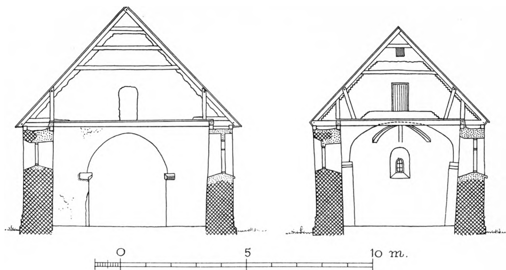
Fig. 4—5. Torsted. Snit gennem Skib og Kor. 1:150. Maalt af Jens Foged 1940. (C. G. Schultz 1941) (S. 400).
