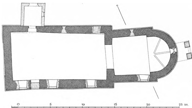
Fig. 2. Vang. Plan. 1:300. Maalt af C. G. Schultz 1937.
