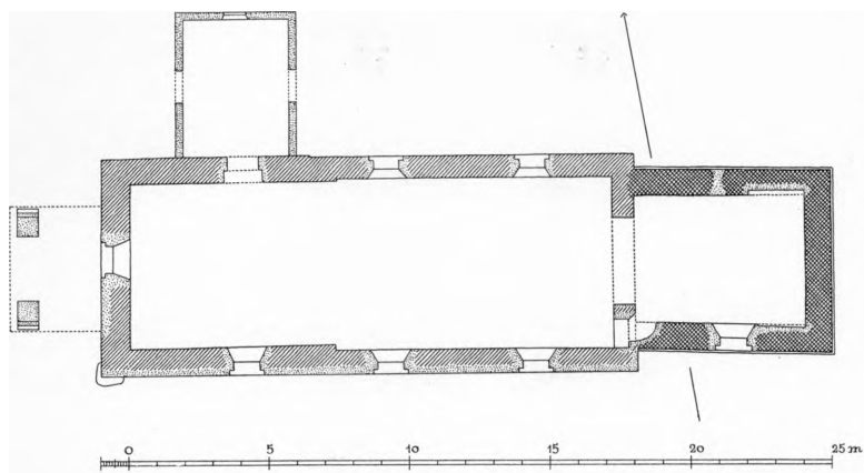
Fig. 2. Janderup. Plan. 1:300. Maalt af C. G. Schultz 1937.
