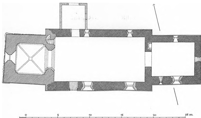
Fig. 2. Sønderhåa. Plan. 1:300. Maalt af C. G. Schultz 1937.
