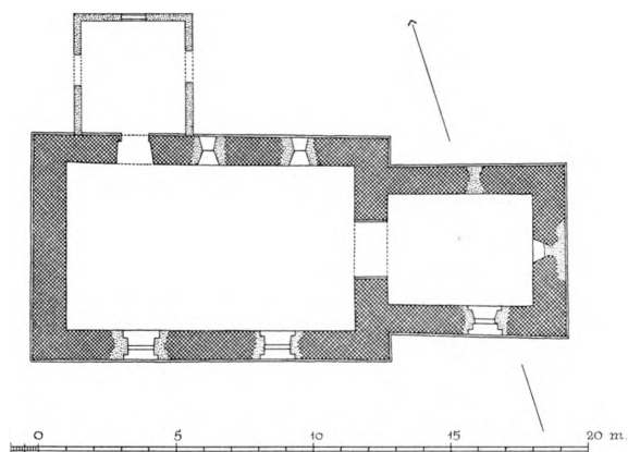
Fig. 2. Haring. Plan. 1:300. Maalt af C. G. Schultz 1937.
