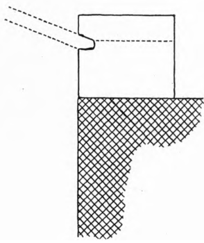
Fig. 5. Karby. Middelalderlig Murrem over Korets Nordmur. 1 : 10 (S. 837).
