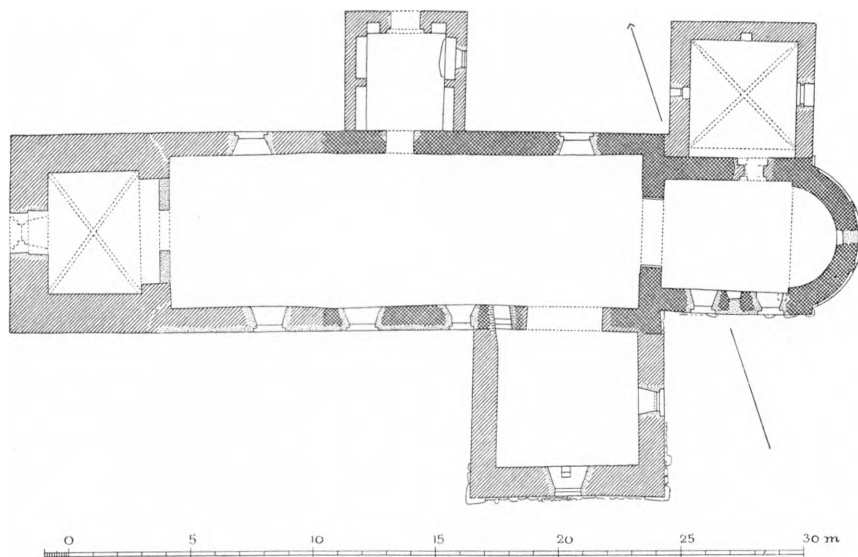
Fig. 2. Karby. Plan. 1 : 300. Maalt af C. G. Schultz 1940.
