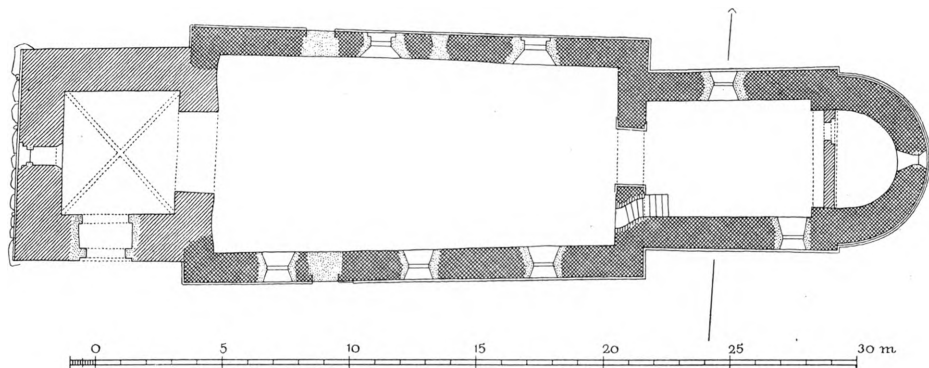
Fig. 2. Hvidbjerg. Plan. 1:300. Maalt af C. G. Schultz 1940.
