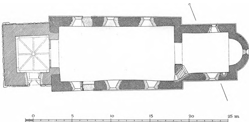
Fig. 2. Ø.-Assels. Plan. 1:300. Maalt af C. G. Schultz 1940.
