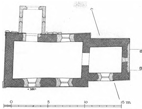
Fig. 2. Ø.-Jølby. Plan. 1:300. Maalt af C. G. Schultz 1940.
