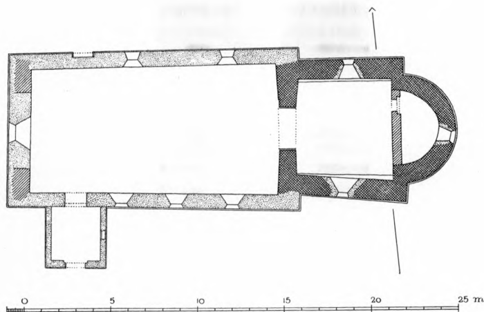
Fig. 2. Sundby. Plan. 1:300. Maalt af G. G. Schultz 1940.
