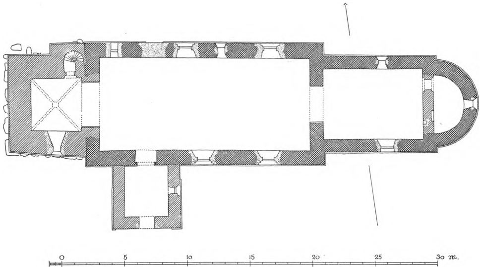
Fig. 2. Sejerslev. Plan. 1:300. Maalt af C. G. Schultz 1939.
