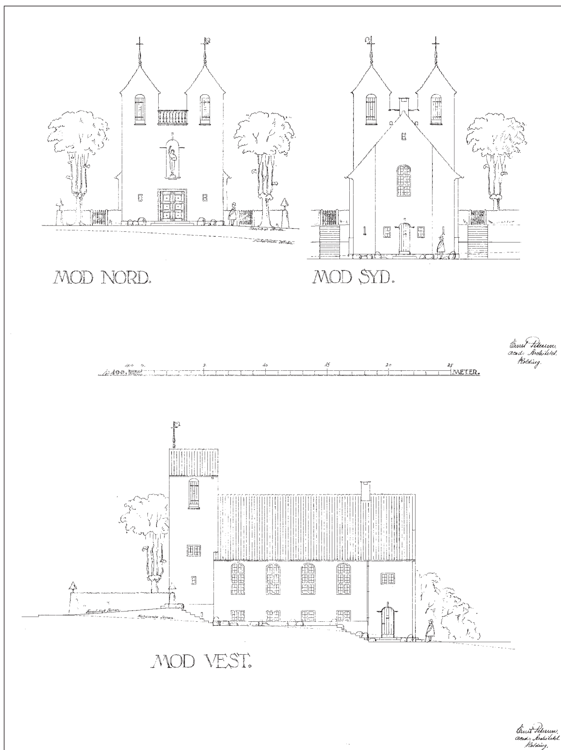
Fig. 4. Forslag til kirken ved Ernst Petersen. Opstalter. 1:300. Tegninger (1930) i Kolding Stadsarkiv. – Proposal for the church by Ernst Petersen. Elevations.
