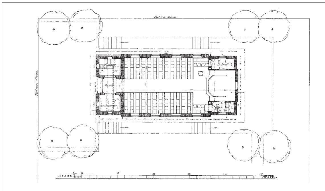
Fig. 3. Forslag til kirken ved Ernst Petersen. Plan. 1:300. Tegning (1930) i Kolding Stadsarkiv. – Proposal for the church by Ernst Petersen. Plan.
