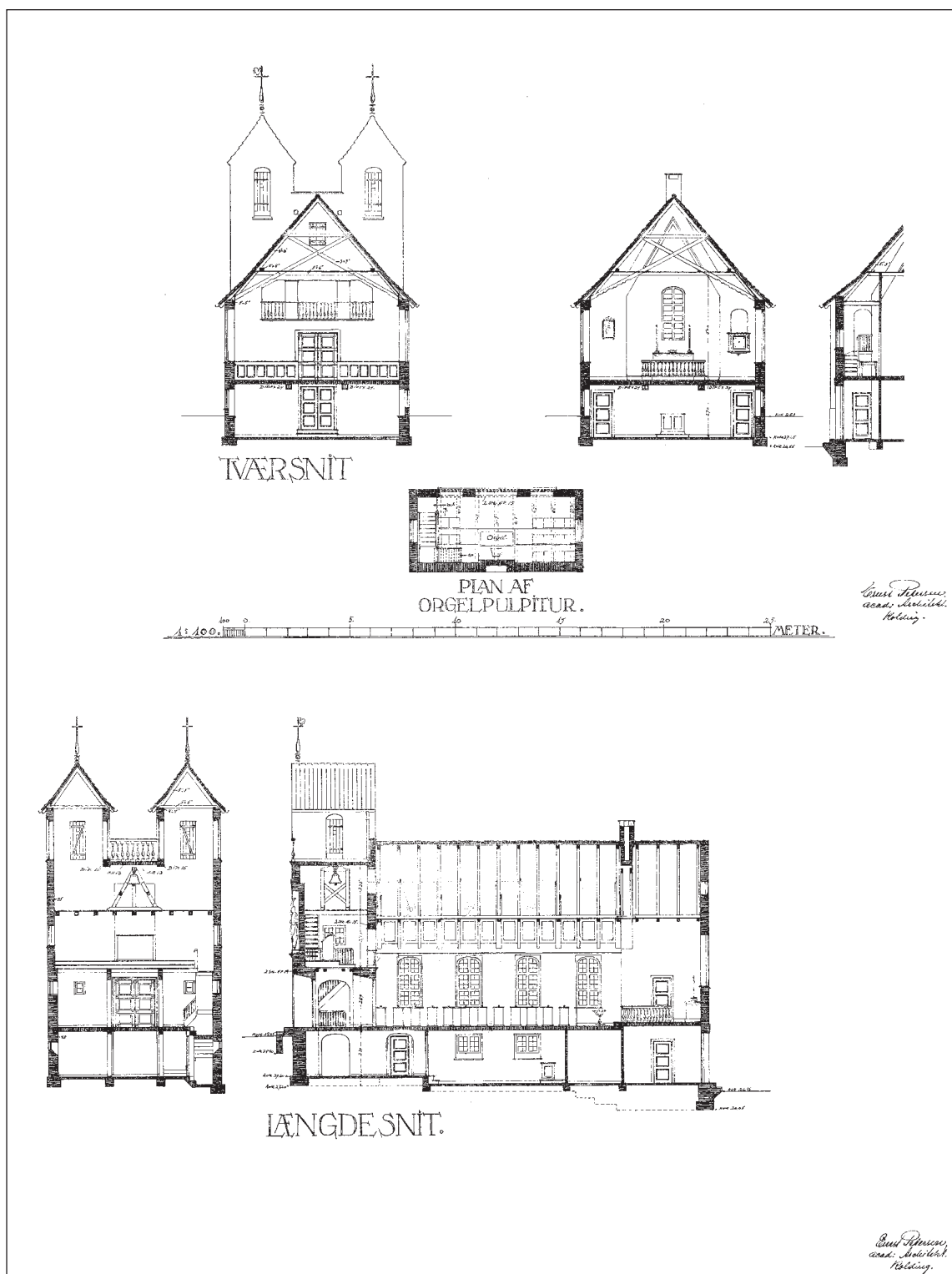
Fig. 5. Forslag til kirken ved Ernst Petersen. Snit. 1:300. Tegninger (1930) i Kolding Stadsarkiv. – Proposal for the church by Ernst Petersen. Sections.
