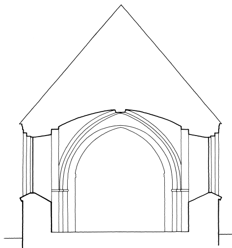
Fig. 5. Tværsnit gennem koret set mod vest. Korbuen havde endnu bevaret rester af \ddagger kragbånd (s. 1350). 1:150. Målt af H. C. Amberg 1902, og tegnet af Merete Rude 2011. – Cross-section through the chancel seen towards the west. The chancel arch still had remains of \ddagger corbelling preserved.
