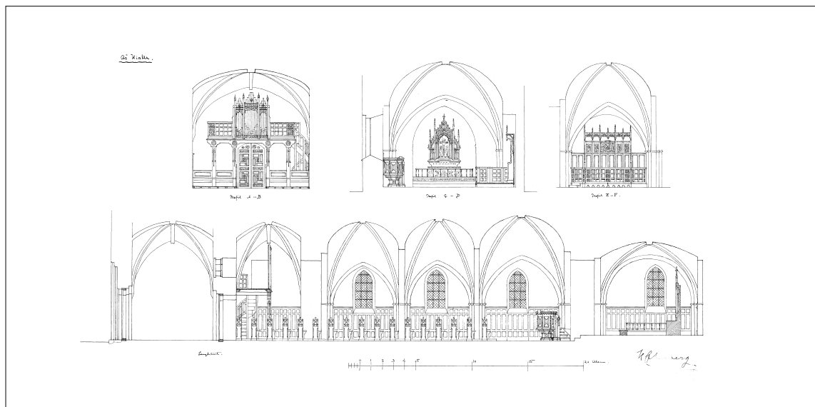
Fig. 15. H. C. Ambergs forslag 1902 til kirkens restaurering, nyt inventar (s. 1355, 1358) og nyt tårn (s. 1356). Tvær-snit og længdesnit, 1:300. – H. C. Amberg's proposal in 1902 for the restoration of the church, new furnishings and a new tower. Cross-section and longitudinal section.
