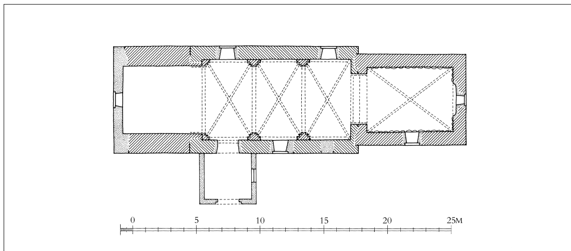
Fig. 4. Grundplan. 1:300. Tegnet af Merete Rude 2011 efter opmåling ved arkitektfirmaet Vilhelmsen, Marxen & Bech-Jensen 2001, suppleret af NJP. – Ground plan.
