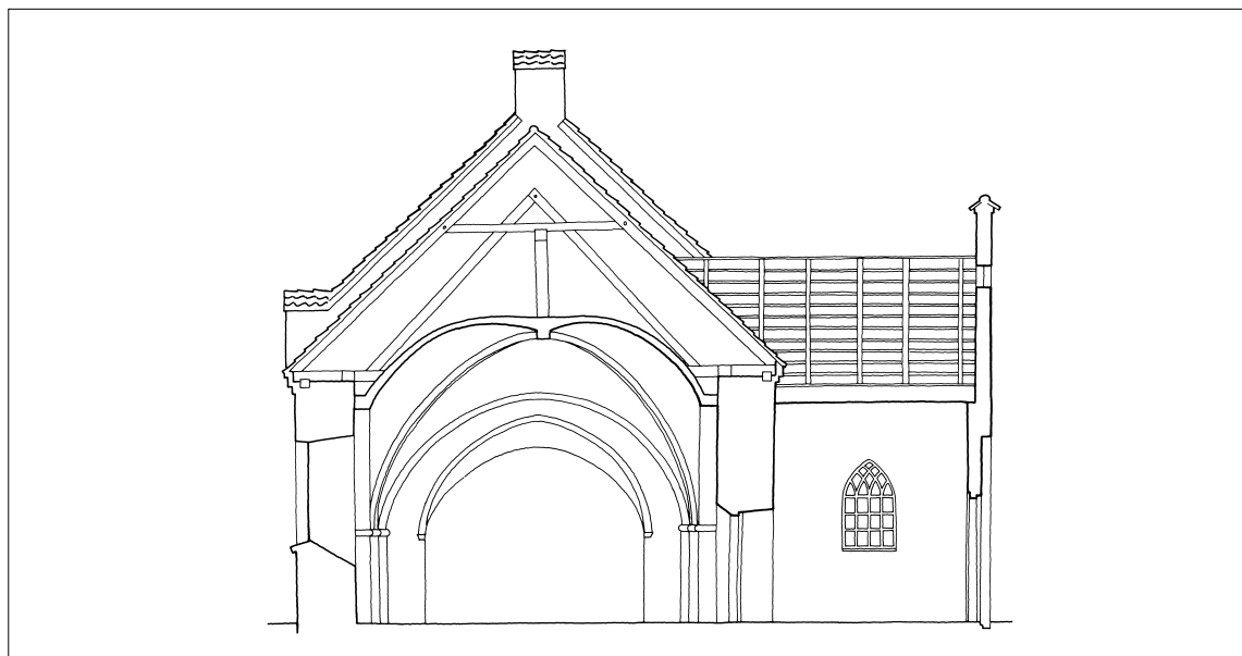
Fig. 5. Tværsnit af skib og våbenhus set mod øst. 1:150. Tegnet af Merete Rude 2011 efter opmåling ved arkitektfirmaet Vilhelmsen, Marxen & Bech-Jensen 2001. – Cross-section of nave and porch seen towards the east.
