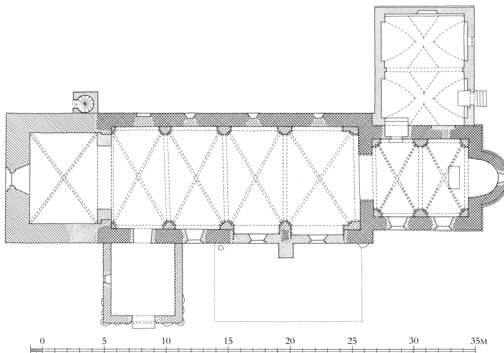
Fig. 5. Grundplan. 1:300. Efter opmåling af Viggo Norn 1941, suppleret af NJP. Tegnet af Merete Rude 2011. – Ground plan.
