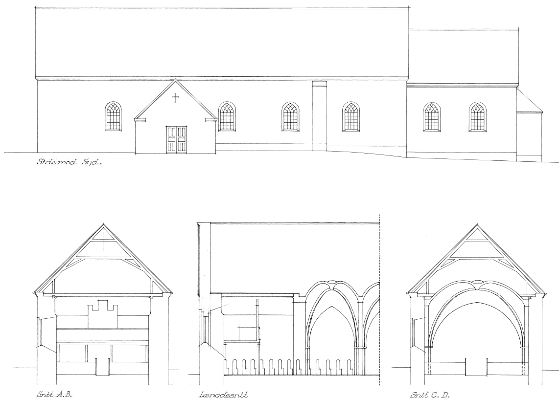
Fig. 8. Kirken før tårnets genopførelse 1943. Opstalt af sydside, tværsnit gennem tårnunderdel og skib, set mod vest, og længdesnit af kirkens vestre del set mod nord. 1:300. Opmåling af Viggo Norn 1941. – The church before the rebuilding of the tower in 1943. Elevation of south side, cross-section through lower tower and nave, seen towards the west, and longitudinal section of the western part of the church, seen towards the north.
