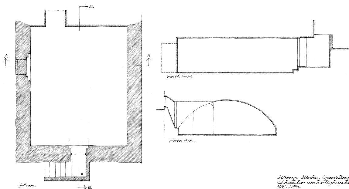
Fig. 13. Hvælvet krypt under adeligt gravkapel, 1670 (s. 1416). Plan og snit, målt og tegnet af Ebbe C. Norn 1961. 1:150. Syd opad. I kirkens arkiv. – Vaulted crypt beneath aristocratic sepulchral chapel, 1670. Plan and section.
