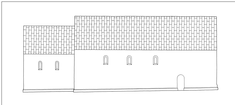
Fig. 8. Den romanske kirke. Opstalt af nordside. Rekonstruktion ved NJP, tegnet af Merete Rude 2011. 1:300. – The Romanesque church. Elevation of north side. Reconstruction.
