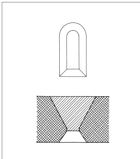
Fig. 9. Romansk vindue i skibets nordside, det midterste (s. 1465). Plansnit og opstalt set udefra. Skitse-mæssig opmåling ved NJP, tegnet af Merete Rude 2011. 1:50. – Romanesque window in north side of nave, middle. Plan section and elevation seen from the outside.
