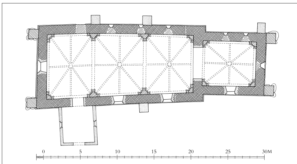
Fig. 6. Grundplan 1:300. Efter opmåling af arkitektfirmaet Hans Vinther, Holger Sørensen & R. Roldsgaard 1961, suppleret af NJP. Tegnet af Merete Rude 2011. – Ground plan.
