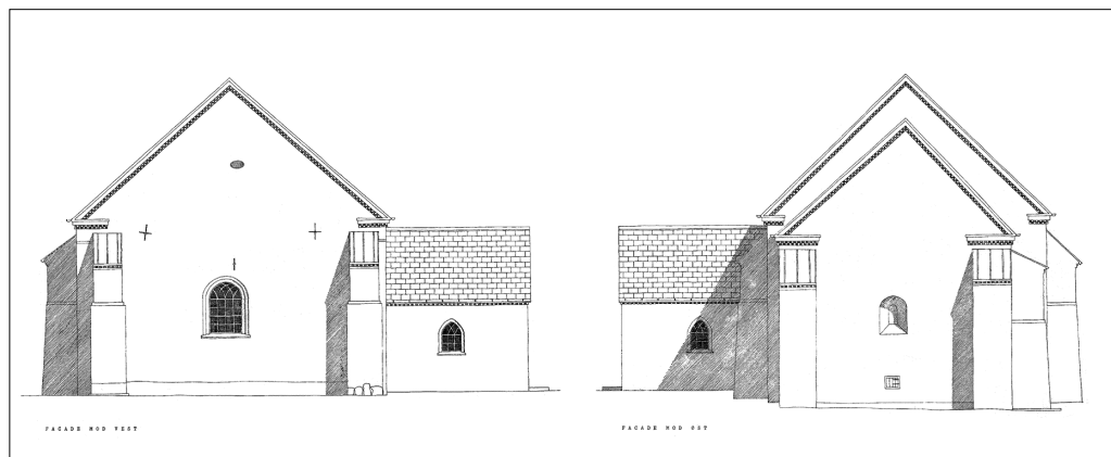
Fig. 7. Opstalt af vest- og østside 1:300. Målt og tegnet af arkitektfirmaet Hans Vinther, Holger Sørensen & R. Roldsgaard 1961. – Elevation of west and east side.
