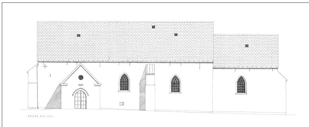
Fig. 5. Opstalt af sydside 1:300. Målt og tegnet af arkitektfirmaet Hans Vinther, Holger Sørensen & R. Roldsgaard 1961. – Elevation of south side.
