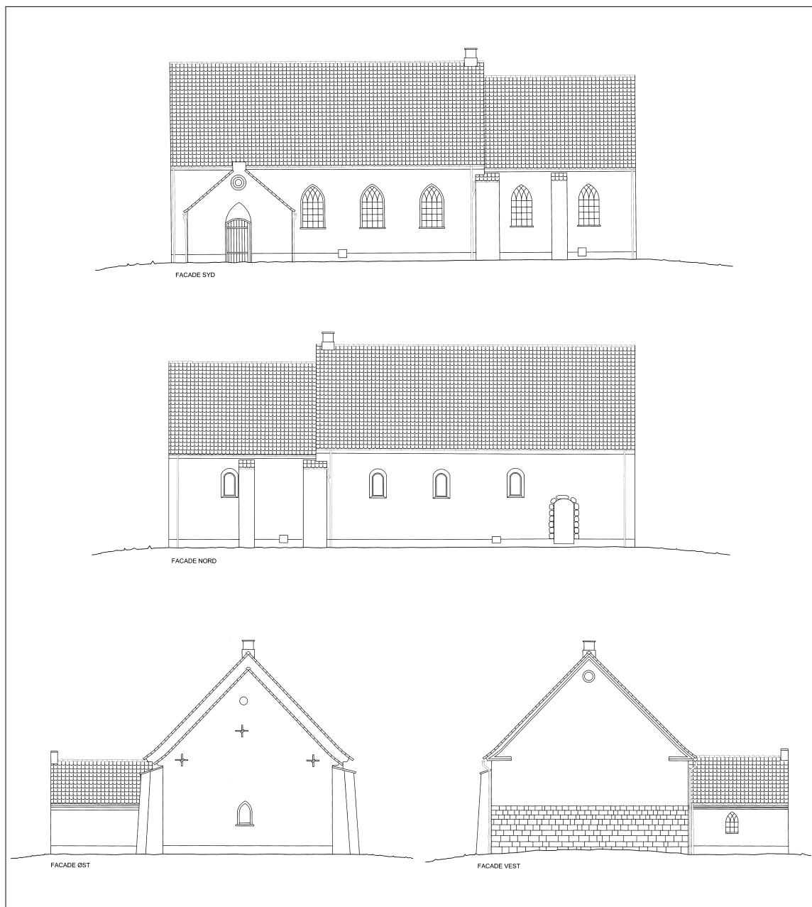
Fig. 9. Opstalter 1:300. Tegnet af arkitektfirmaet Birch & Svenning 2008 efter maskinel opmåling. Den angivne sokkel er en svættet fod. – Elevations.
