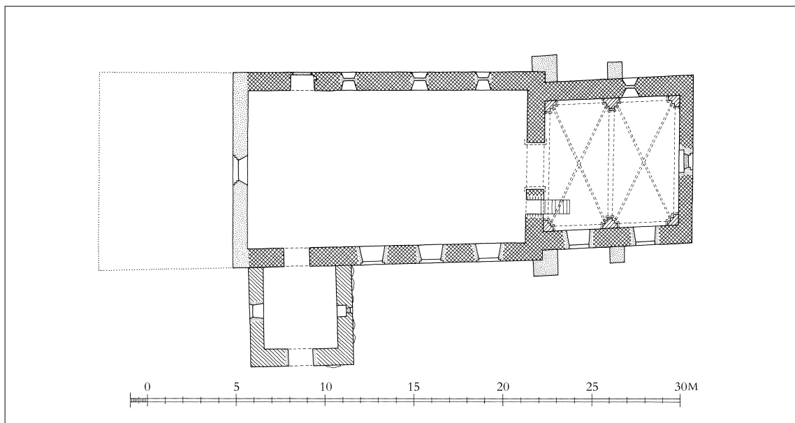
Fig. 7. Grundplan. 1:300. Tegnet af Merete Rude 2011 efter opmåling ved arkitektfirmaet Birch & Svenning 2006, suppleret af NJP. – Ground plan.
