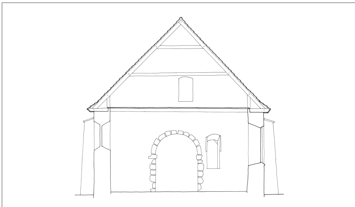
Fig. 8. Tværsnit gennem skibet set mod øst. 1:150. Målt af Anders C. Christensen og Mogens Vedsø 2012, tegnet af sidstnævnte. – Cross-section of nave seen towards the east.
