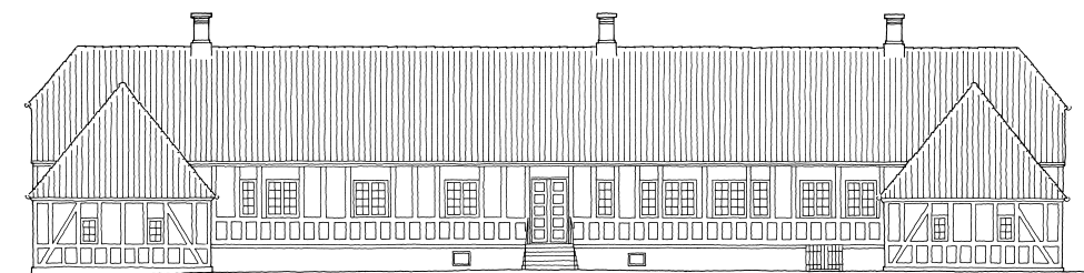
Fig. 4. †Præstegårdens hovedbygning, opført o. 1740 og nedrevet 1936 (s. 1486). Sydsiden set fra gårdspladsen. Målt af Viggo Norn 1935, tegnet af Merete Rude 2011. 1:300. – Main building of rectory, built c. 1740 and demolished in 1936. South side seen from courtyard.
