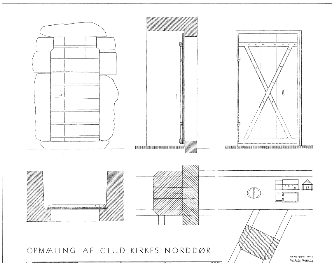
Fig. 10. Norddøren efter genåbningen 1948, udvendig opstalt, plan og tværsnit set mod vest (s. 1489). I åbningen ses den delvis rekonstruerede \star dørfloj fra o. 1650-1700, nu i Horsens Museum (s. 1510). Målt og tegnet af Vilhelm Wittrup 1948. 1:50. – North door after re-opening, 1948, exterior elevation, plan and cross-section seen towards the west. In the opening the partly reconstructed \star door leaf from c. 1650-1700 can be seen.
