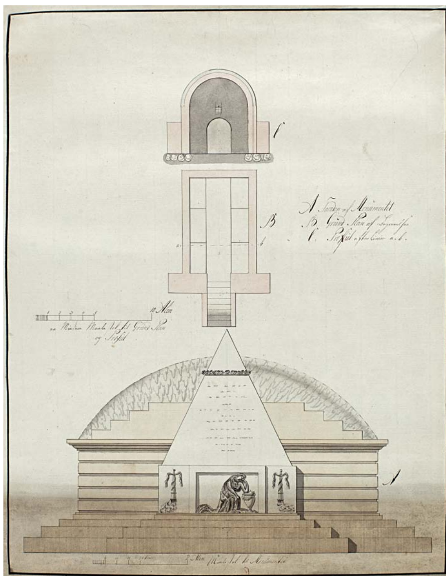
Fig. 39. Mausoleum, o. 1803, for Lars Thygeson til Bygholm og hans familie, tegning til monumentet af bygmester Johan Jørgen Høffner i Horsens (s. 1577-78, jf. fig. 38). Opstalt 1:50; plan og snit 1:200. I Landsarkivet for Fyn. — Mausoleum, c. 1803, for Lars Thygeson of Bygholm and his family, drawing for the monument by the master-builder Johan Jørgen Høffner in Horsens.
