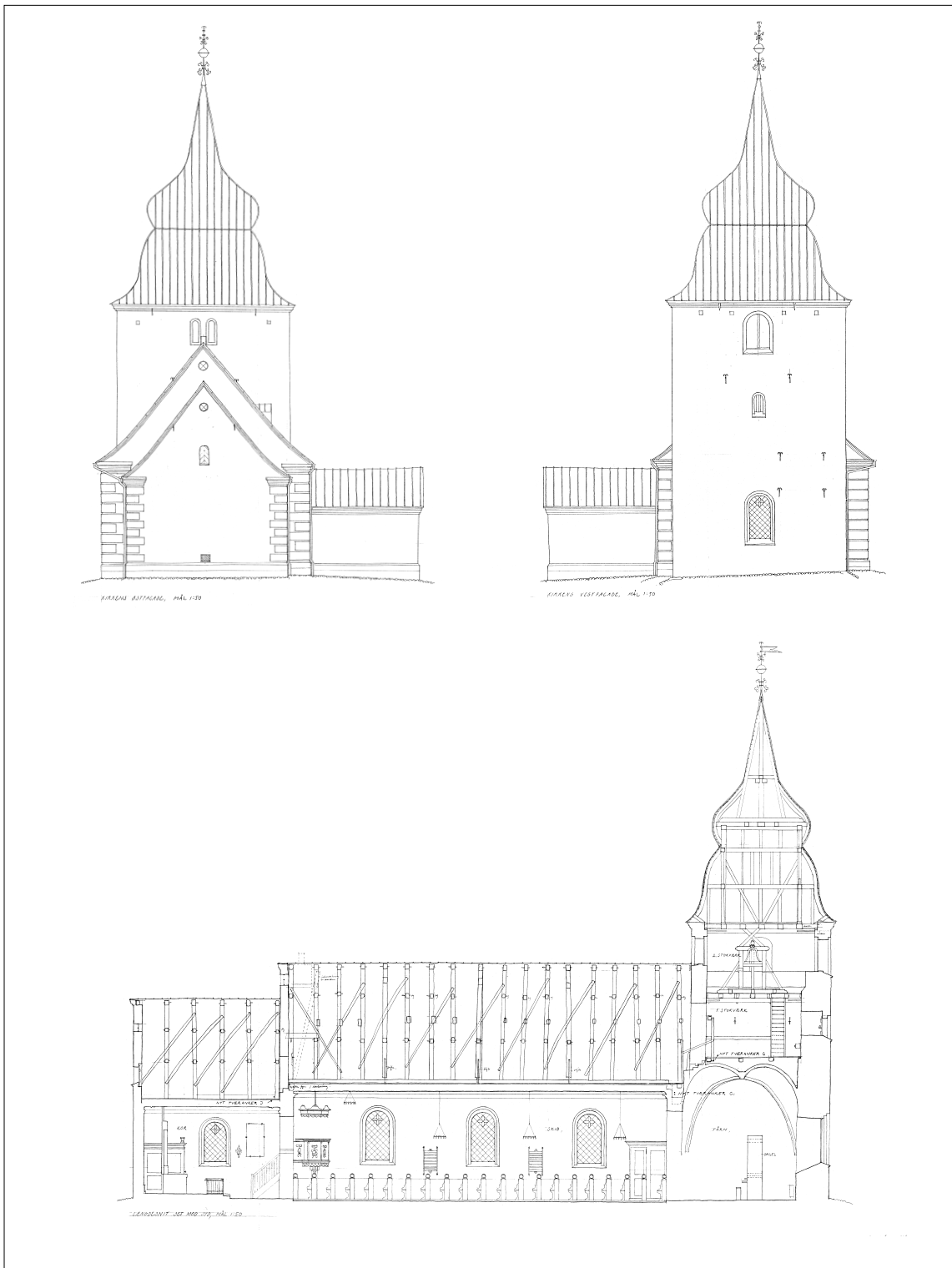
Fig. 7b. Opstalter af øst- og vestfacaden. Længdesnit set mod syd. 1:300. Målt og tegnet af Per Kristensens Tegnastue 1990. – Elevations of the east and west facade. Longitudinal section seen towards the south.
