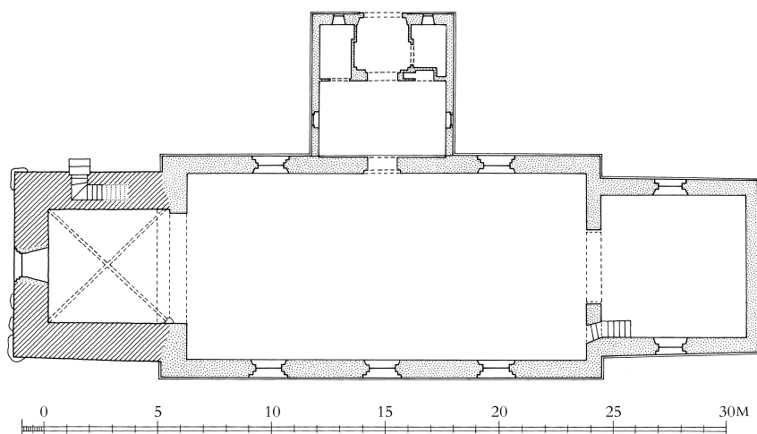
Fig. 6. Grundplan. 1:300. Tegnet af Merete Rude 2012 efter opmåling af arkitektfirmaet Per Kristensens Tegnstue 1990, suppleret af NJP. – Ground plan .
