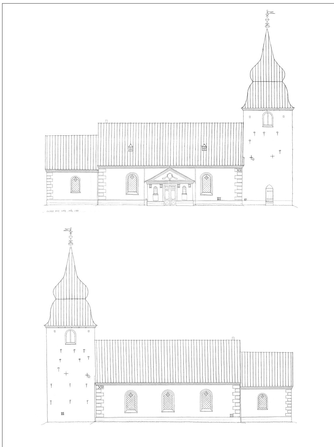
Fig. 7a. Opstalter af nord- og sydfacaden. 1:300. Målt og tegnet af Per Kristensens Tegnestue 1990. — Elevations of the north and south facade.
