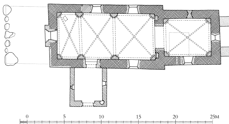
Fig. 5. Grundplan. 1:300. Tegnet af Merete Rude 2012 efter opmåling af Inger og Johannes Exners Tegnestue 1968, suppleret af NJP. – Ground plan.
