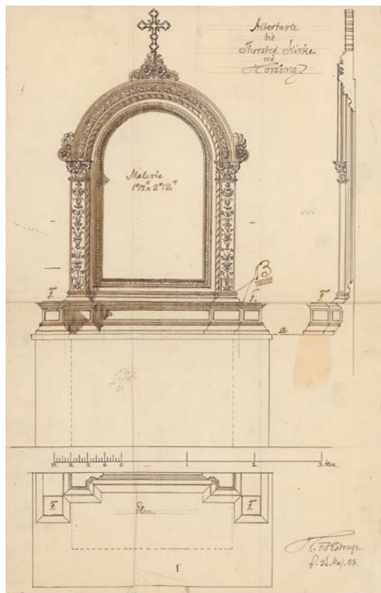
Fig. 16. *Altartavle, 1884, tegning ved Hector Estrup 1883 (s. 1611-12). 1:50. I Horsens Museum. – *Altarpiece, 1884.
