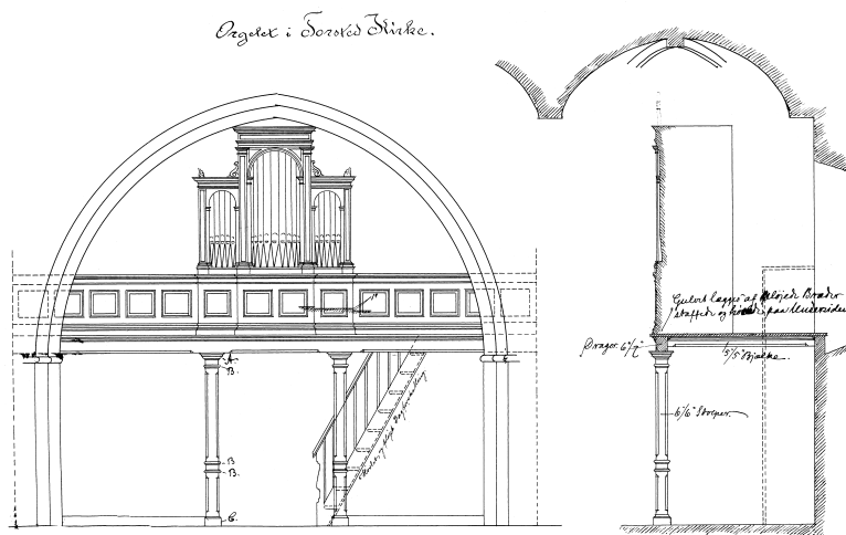
Fig. 35. Tegning af orgelpulpitur og -facade (s. 1620) ved Hector Estrup, 1886. 1:100. I Horsens Museum. – Drawing of organ loft and casing.
