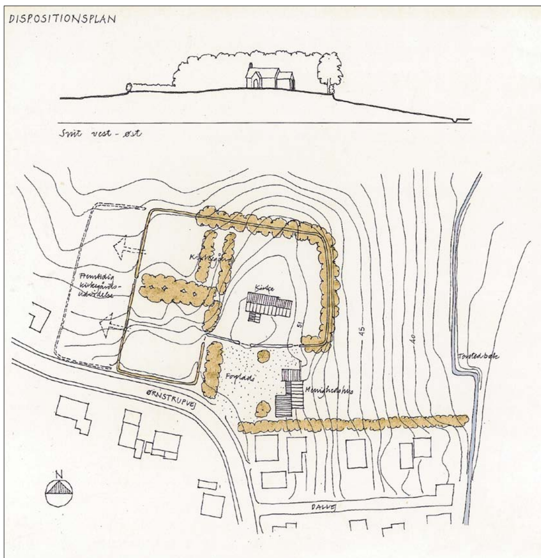
Fig. 3. Dispositionsplan 1979 ved Erik Lerbech-Sørensen's Tegnestue. Tegning i kirkens arkiv. 1:2.000. Forslaget til menighedshus og udvidelse af kirkegården kom ikke til udførelse. – Layout plan, 1979.
