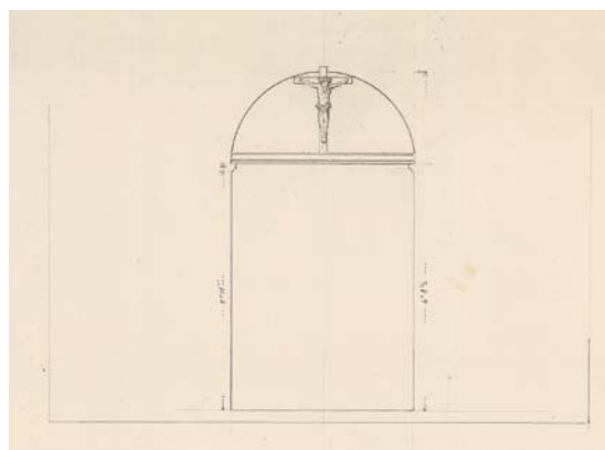
Fig. 7-8. Romansk triumfvæg og \dagger korbue. 1:100. 7. \dagger Korbue og \dagger sidealternicher samt oprindeligt gulvniveau (s. 1602, 1606). Rekonstruktion ved NJP, tegnet af Merete Rude 2012. 8. \dagger Korbuen før udvidelse 1876 (s. 1602) vist med krucifiks fra o. 1475-1500 og \dagger korbeubjælke (s. 1615). Opstalt målt og tegnet af L. A. Winstrup 1875. – Romanesque chancel arch wall and \dagger chancel arch. 7. \dagger Chancel arch and \dagger side altar niches, with original floor level. Reconstruction. 8. \dagger Arch before expansion in 1876, shown with crucifix from c. 1475-1500 and \dagger chancel arch beam. Elevation.
