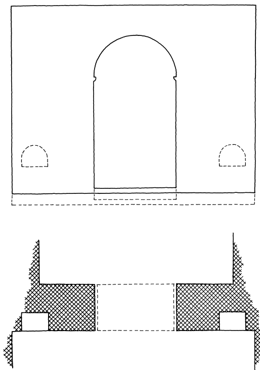
Fig. 7-8. Romansk triumfvæg og \dagger korbue. 1:100. 7. \dagger Korbue og \dagger sidealternicher samt oprindeligt gulvniveau (s. 1602, 1606). Rekonstruktion ved NJP, tegnet af Merete Rude 2012. 8. \dagger Korbuen før udvidelse 1876 (s. 1602) vist med krucifiks fra o. 1475-1500 og \dagger korbeubjælke (s. 1615). Opstalt målt og tegnet af L. A. Winstrup 1875. – Romanesque chancel arch wall and \dagger chancel arch. 7. \dagger Chancel arch and \dagger side altar niches, with original floor level. Reconstruction. 8. \dagger Arch before expansion in 1876, shown with crucifix from c. 1475-1500 and \dagger chancel arch beam. Elevation.
