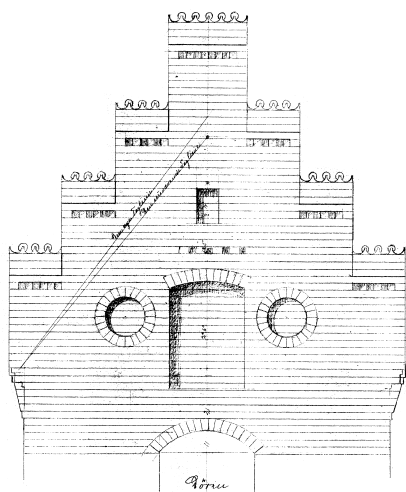
Fig. 7. Forslag til ombygning af våbenhusets gavle ved Carl Kiilsgaard 1913 (s. 1637). Tegning i Landsarkivet. 1:100. – Proposal for rebuilding of porch gable from Carl Kiilsgaard, 1913.
