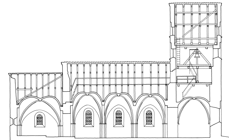
Fig. 3. Længdesnit set mod syd. 1:300. Tegnet af Merete Rude 2012 efter Ebbe C. Norn 1959 og Arkitektfirmaet Vilhelmsen, Marxen & Bech-Jensen 1993. – Longitudinal section seen towards the north.
