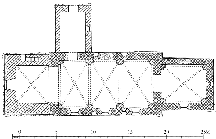
Fig. 4. Grundplan. 1:300. Tegnet af Merete Rude 2012 efter opmåling af Ebbe C. Norn 1959, suppleret af NJP. – Ground plan.
