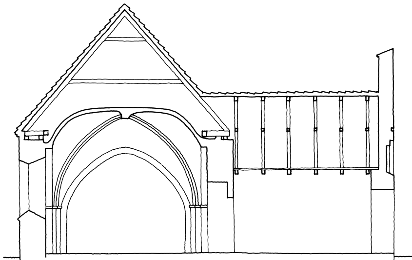
Fig. 5. Tværsnit gennem skib og våbenhus set mod vest. Tegnet af Merete Rude 2012 efter Ebbe C. Norn 1959. 1:150. — Cross-section through nave and porch seen towards the west.
