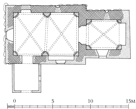
Fig. 3. Grundplan. 1:300. Tegnet af Merete Rude 2013 efter Helge Andreassen 1968, suppleret af Niels Jørgen Poulsen. – Ground plan.
