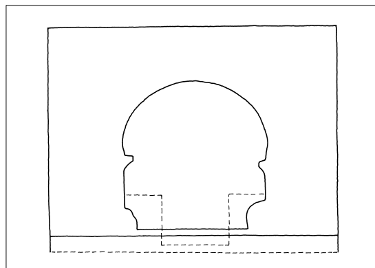
Fig. 6. Romansk triumfvæg med korbue og forslag til †korskranke med en dør i midten (s. 1887). 1:100. Rekonstruktion med oprindeligt gulvniveau ved Niels Jørgen Poulsen, tegnet af Merete Rude 2013. – Romanesque chancel wall with chancel arch and proposal for chancel rail with a door in the middle. Reconstruction with original floor level.
