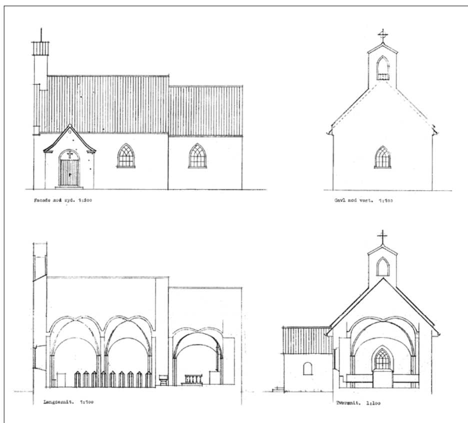
Fig. 5. Opstalter og snit. 1:300. Skitse-mæssig opmåling ved Helge Andreassen 1968. – Elevations and sections.
