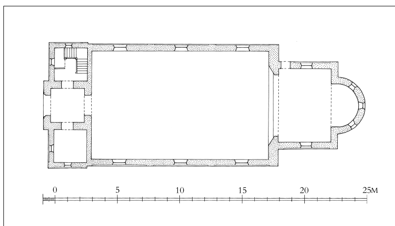
Fig. 3. Grundplan 1:300. Efter opmåling af Kuno og Ejnar N. Mielby, suppleret af Niels Jørgen Poulsen. Tegnet af Merete Rude 2014. – Ground plan.
