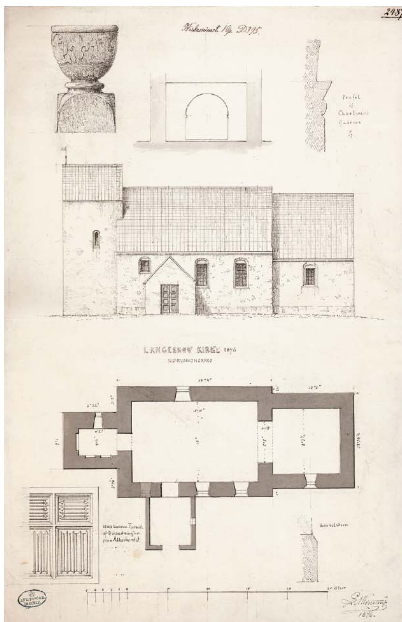
Fig. 8. Den nedrevne \dagger kirke. Plan, opstalt af sydside og tværsnit af skib set mod øst. 1:300. Hertil døbefont (s. 2233) og \dagger alterbordsforside (s. 2225) samt profiler af korbuekragbånd og skråkantsokkel (s. 2220). Målt og tegnet af L.A. Winstrup 1876. — The demolished \dagger church. Plan, elevation of south side and cross-section of nave looking east. Font and \dagger Communion table frontal, and profiles of chancel arch corbelling and bevelled footing.
