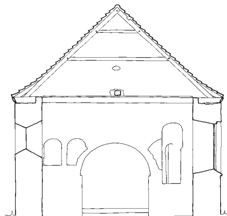
Fig. 7. Tværsnit gennem skibet set mod øst. 1:150. Målt og tegnet af Anders C. Christensen 2016. – Section through nave seen towards the east.
