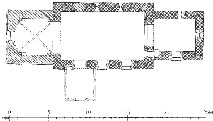
Fig. 5. Grundplan 1:300. Målt af Kuno Mielby 2010, suppleret af Jakob Kieffer-Olsen og tegnet af Anders C. Christensen 2016. – Ground plan.
