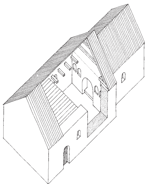
Fig. 6. Rekonstruktion af skib og kor med triumfmur og styrtrum. 1:300. Tegnet af Thomas Bertelsen 2016. – Reconstruction of nave and chancel with triumphal wall and upper storey.
