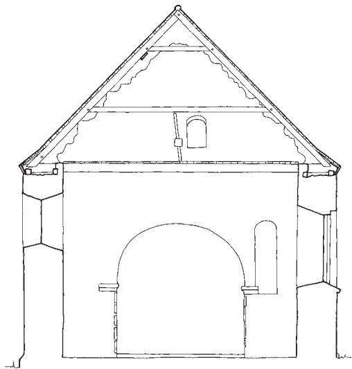
Fig. 6. Tværsnit gennem skibet set mod øst. 1:150. Målt og tegnet af Anders C. Christensen 2016. – Section of nave seen towards the east.
