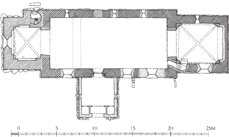
Fig. 7. Grundplan. 1:300. Målt af Birch & Svenning 1998, suppleret af Jakob Kieffer-Olsen og tegnet af Anders C. Christensen 2016. – Ground plan.
