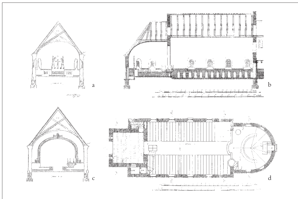
Fig. 3a-d. Tegninger af kirken. 1:300. a. Tværsnit af koret set mod øst. b. Længdesnit gennem kor og skib set mod syd. c. Tværsnit af skibet set mod øst. d. Grundplan. Tegninger ved N. Christof Hansen 1913. I Vejle Stadsarkiv. – Drawings of church. a. Cross section of chancel looking east. b. Longitudinal section of chancel and nave looking south. c. Cross section of nave looking east. d. Ground plan.
