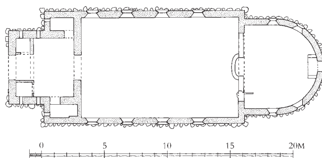
Fig. 4. Grundplan. 1:300. Tegnet af Anders C. Christensen 2016 på grundlag af tegning ved N. Christof Hansen 1913. – Ground plan.
