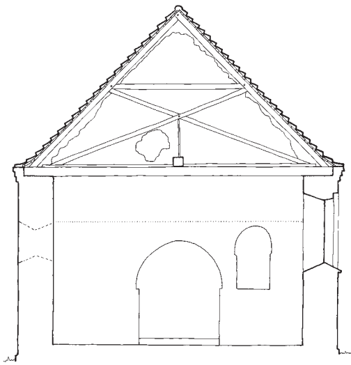
Fig. 5. Tværsnit gennem skib set mod øst. 1:150. Målt af Anders C. Christensen og Jakob Kieffer-Olsen, tegnet af Anders C. Christensen 2016. – Cross-section through nave looking east.
