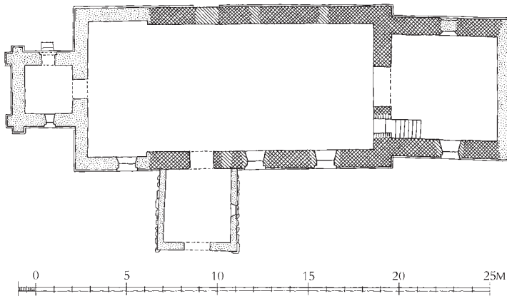
Fig. 6. Grundplan. 1:300. Målt af Ebbe Lehn Petersen 1982, suppleret af Jakob Kieffer-Olsen og tegnet af Anders C. Christensen 2016. – Ground plan.
